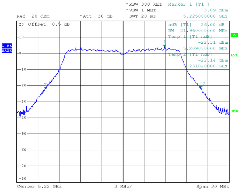
Antenna A - 802.11a – 5220MHz
