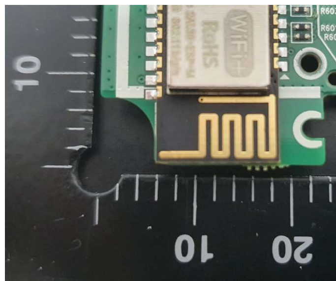
Antenna
