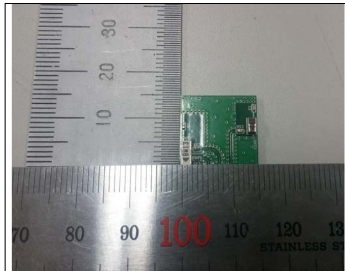
<Ant: BT, WLAN>
