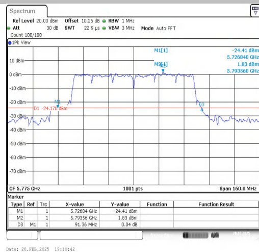
11AC80SISO-Ant1-5775
