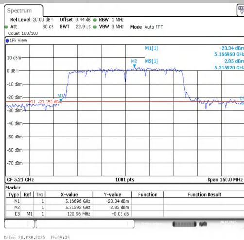
11AC80SISO-Ant1-5210
