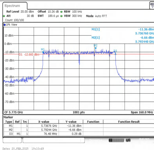
11AC80SISO-Ant1-5775-PASS
