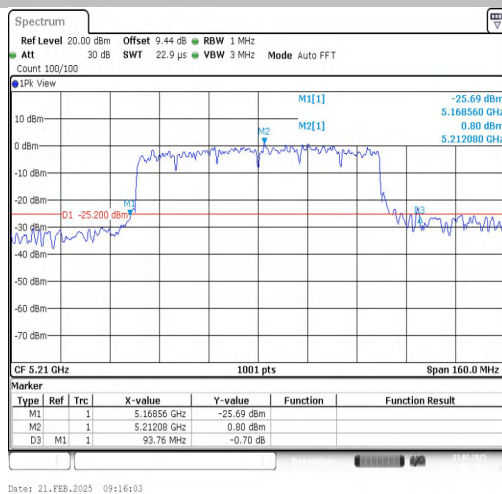
11AX80SISO-Ant1-5210
