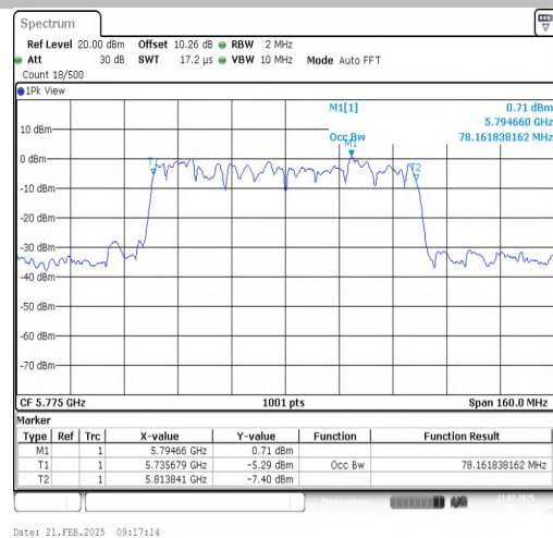
11AX80SISO-Ant1-5775
