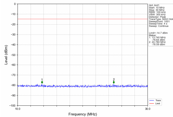
10MHz-30MHz
