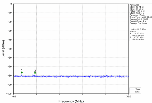
10MHz-30MHz
