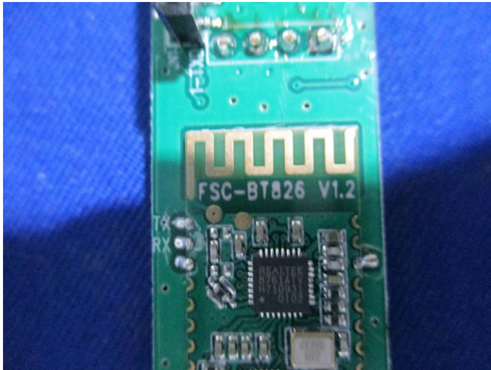
RF ANT
