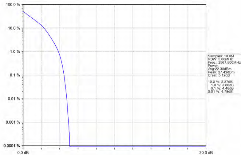
Band7_5MHz_QPSK_HCH_2567.5MHz_RB_25_0_NTNV
