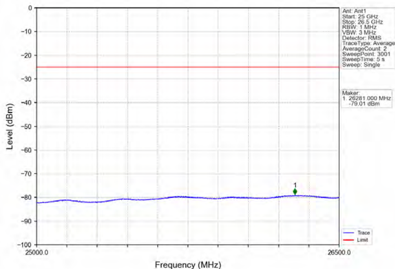
Band7 10MHz QPSK MCH 2535MHz RB 1 0 NTN
