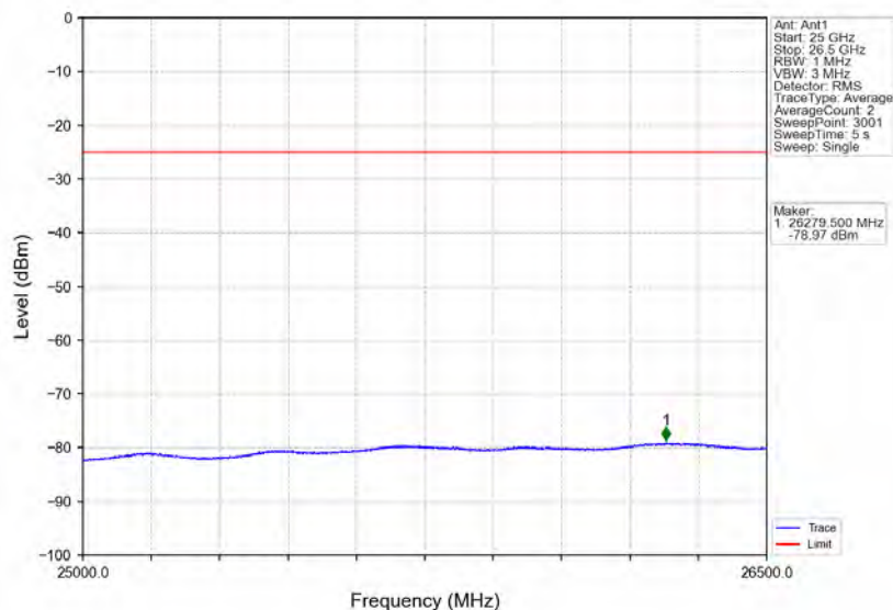
Band7_10MHz_QPSK_LCH_2505MHz_RB_1_0_NTNV
