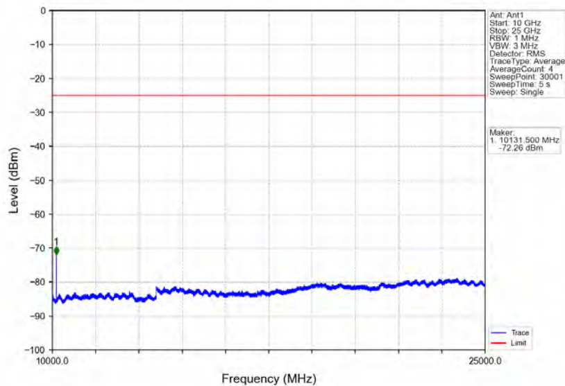
Band7_5MHz_QPSK_MCH_2535MHz_RB_1_0_NTNV
