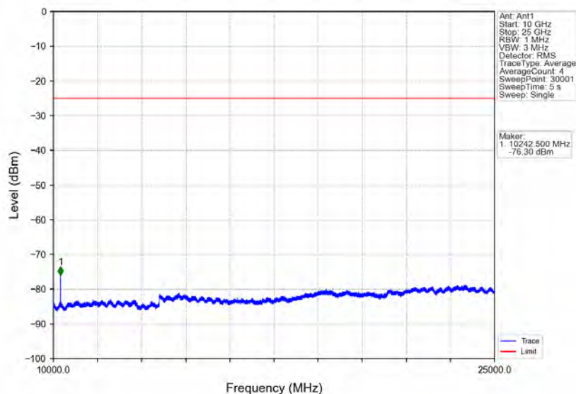
Band7_10MHz_QPSK_HCH_2565MHz_RB_1_0_NTNV
