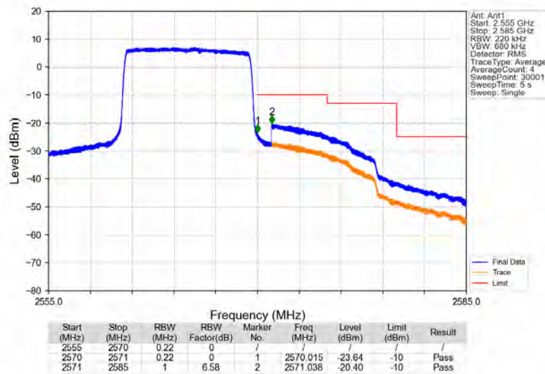
Band7 10MHz QPSK HCH 2565MHz RB 50 0 NTNV
