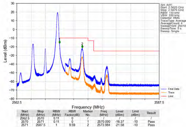
Band7_5MHz_QPSK_HCH_2567.5MHz_RB_1_24_NTNV
