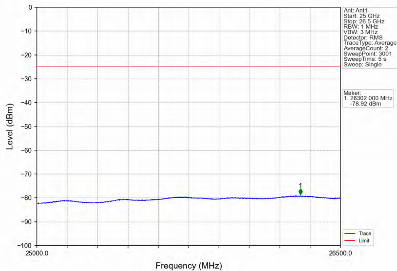
Band7 20MHz QPSK HCH 2560MHz RB 1 99 NTNV
