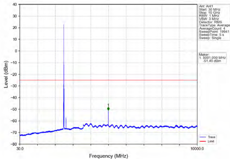
Band7 10MHz 16QAM LCH 2505MHz RB 1 0 NTNV
