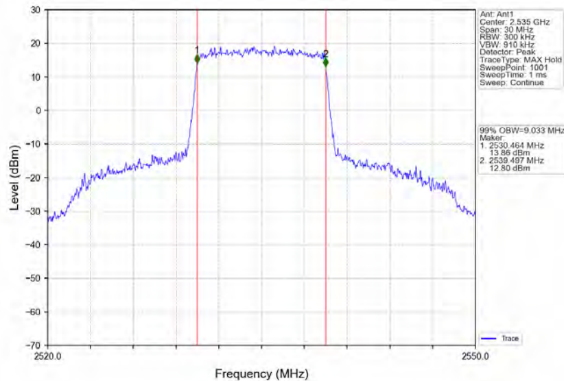
Band7_10MHz_QPSK_MCH_2535MHz_RB_50_0_NTNV
