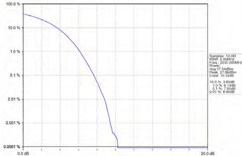
Band7 20MHz 16QAM MCH 2535MHz RB 100 0 NTNV
