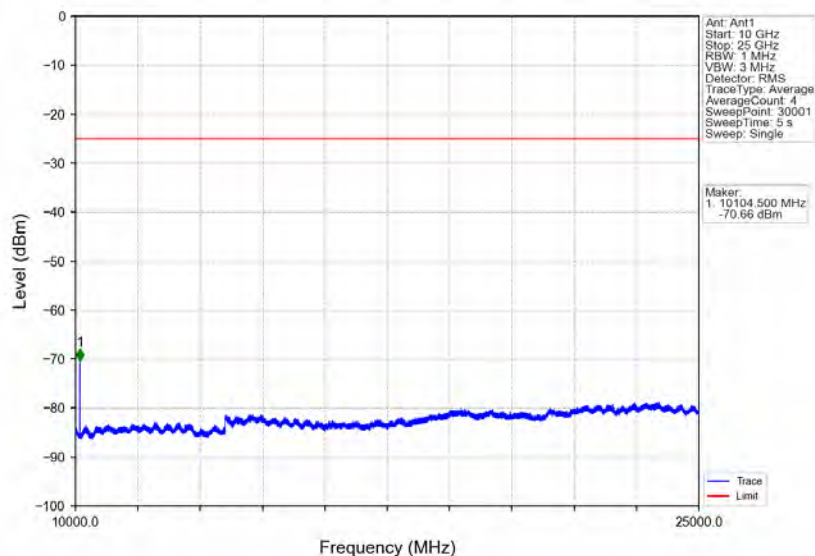
Band7 20MHz 16QAM MCH 2535MHz RB 1 0 NTNV
