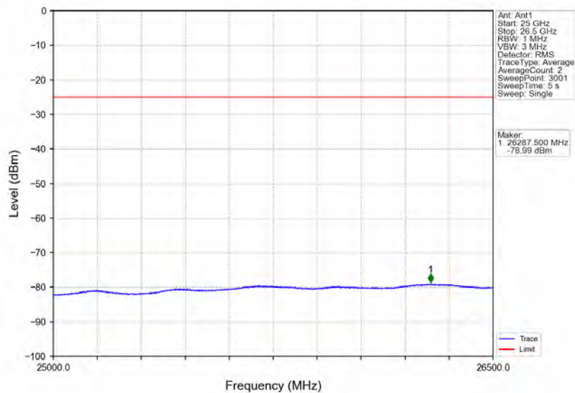
Band7_5MHz_QPSK_HCH_2567.5MHz_RB_1_24_NTNV
