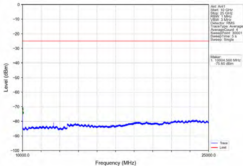
Band7_20MHz_QPSK_LCH_2510MHz_RB_1_0_NTNV
