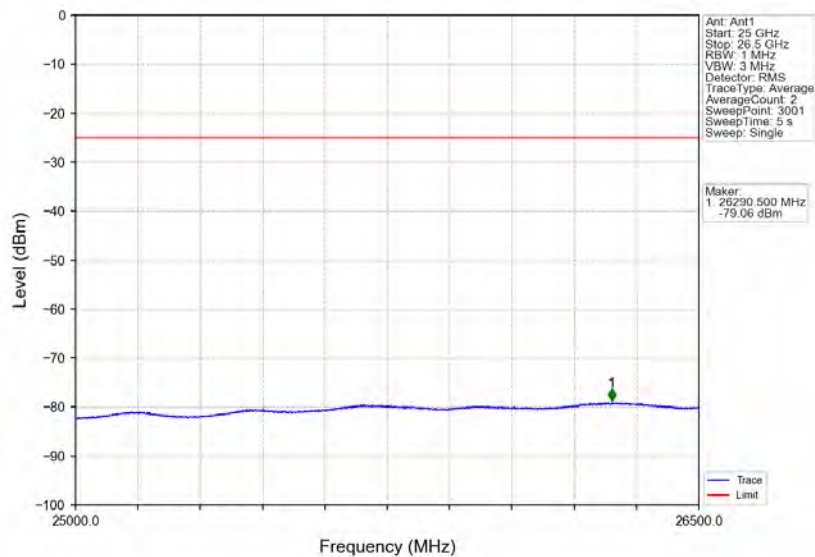
Band7_15MHz_QPSK_HCH_2562.5MHz_RB_1_74_NTNV
