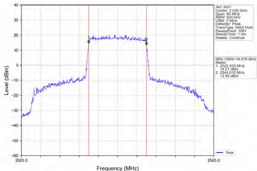
Band7_20MHz_QPSK_MCH_2535MHz_RB_100_0_NTNV
