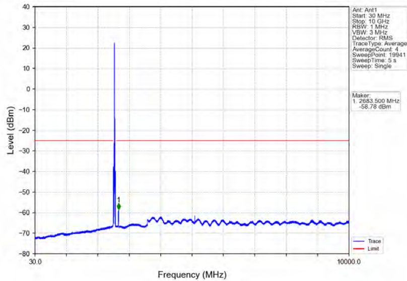
Band7_20MHz_QPSK_HCH_2560MHz_RB_1_0_NTNV
