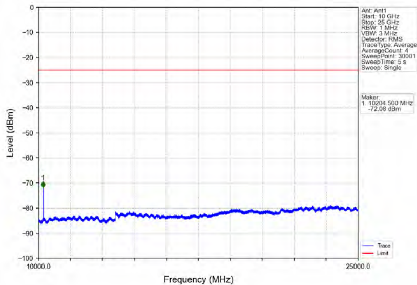
Band7_20MHz_QPSK_HCH_2560MHz_RB_1_0_NTNV
