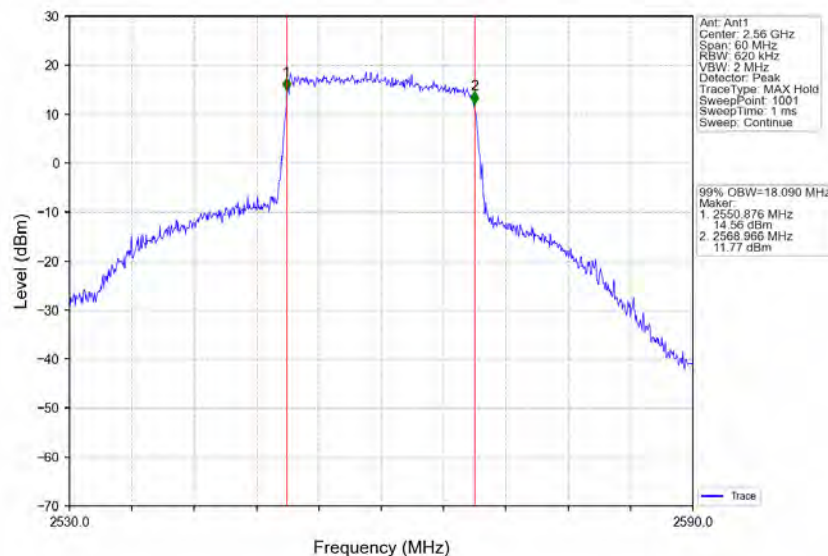
Band7 20MHz 16QAM HCH 2560MHz RB 100 0 NTNV
