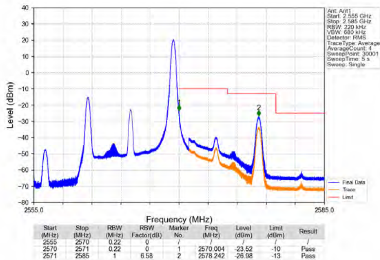
Band7 10MHz QPSK HCH 2565MHz RB 1 49 NTNV
