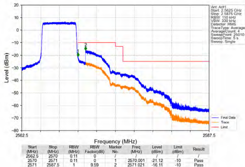
Band7_5MHz_QPSK_HCH_2567.5MHz_RB_25_0_NTNV
