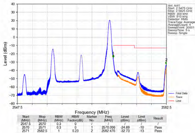
Band7_15MHz_QPSK_HCH_2562.5MHz_RB_1_74_NTNV
