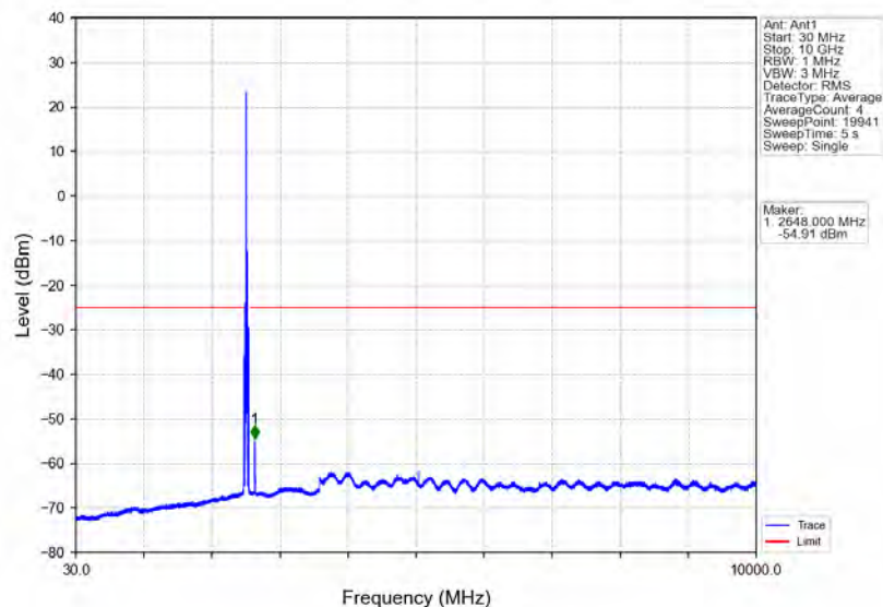
Band7_20MHz_QPSK_MCH_2535MHz_RB_1_0_NTNV
