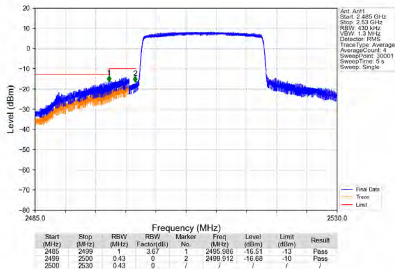
Band7_20MHz_QPSK_LCH_2510MHz_RB_100_0_NTNV
