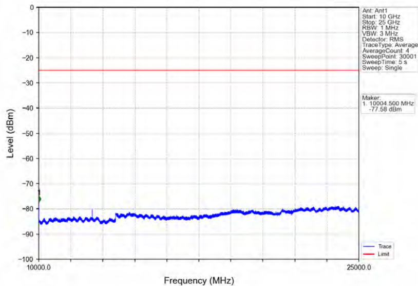
Band7 20MHz 16QAM LCH 2510MHz RB 1 0 NTNV
