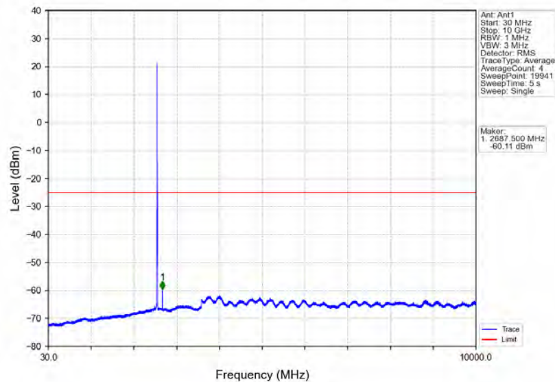
Band7 5MHz QPSK HCH 2567.5MHz RB 1 0 NTN
