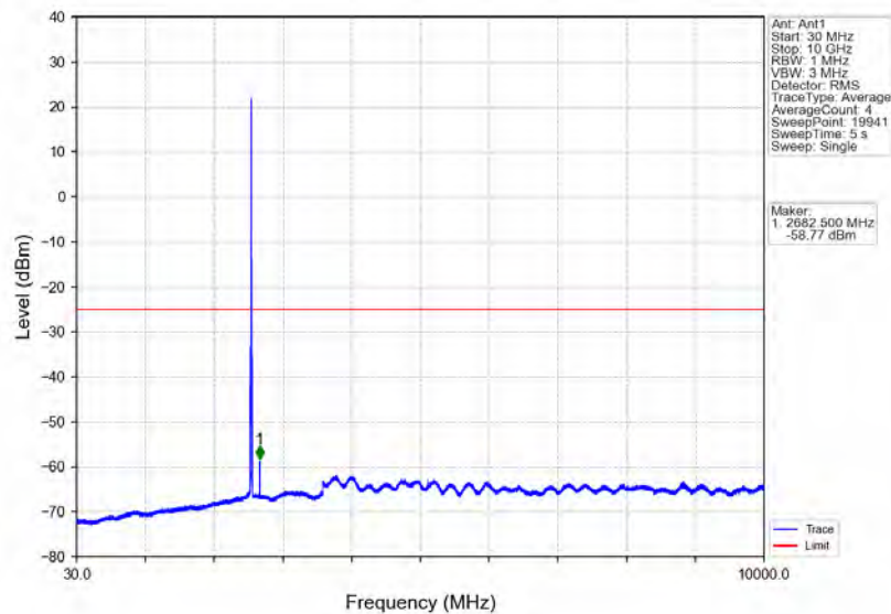
Band7_10MHz_QPSK_HCH_2565MHz_RB_1_0_NTNV
