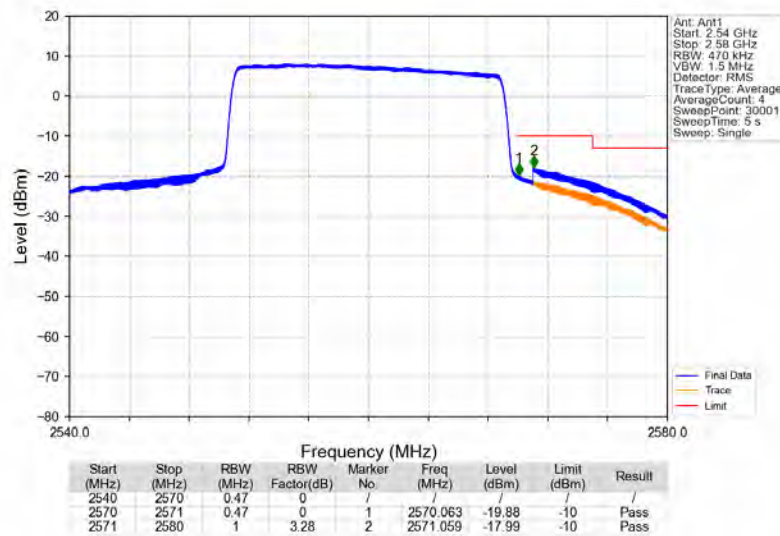
Band7 20MHz QPSK HCH 2560MHz RB 100 0 NTNV
