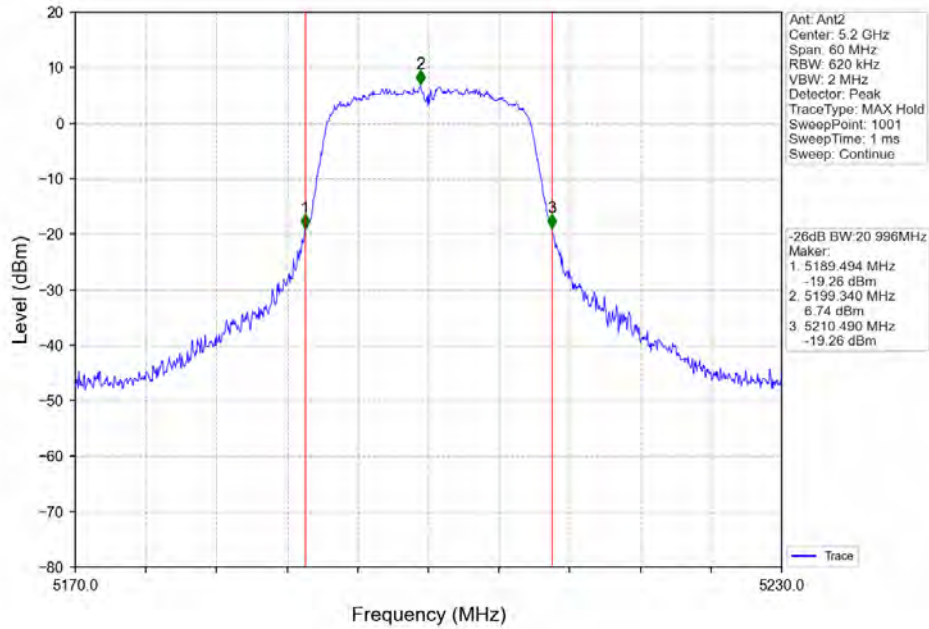
802.11n(HT20)_MCH_5200MHz_Ant2_NTNV
