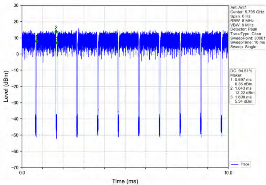
802.11n(HT40)_HCH_5795MHz_Ant1_NTNV
