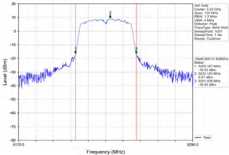
802.11n(HT40)_HCH_5230MHz_Ant2_NTNV
