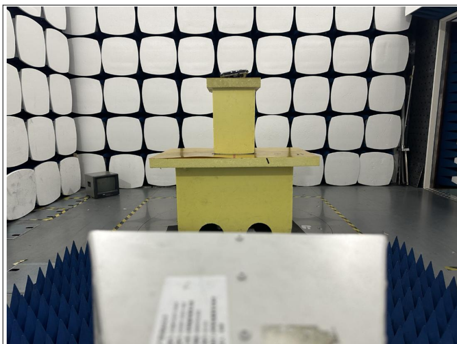
1GHz-18GHz(BT&BLE)
