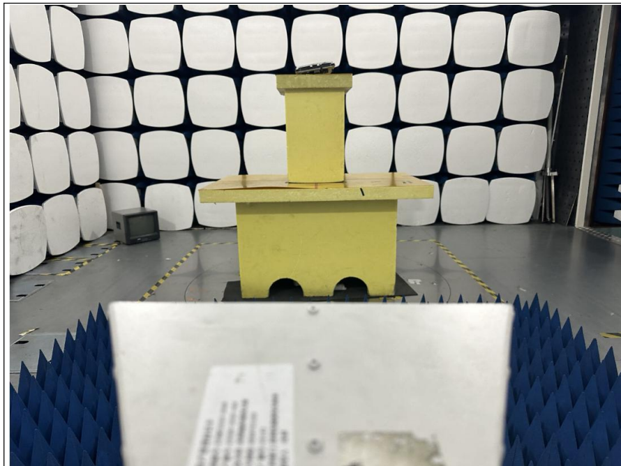
1GHz-18GHz(WiFi)
