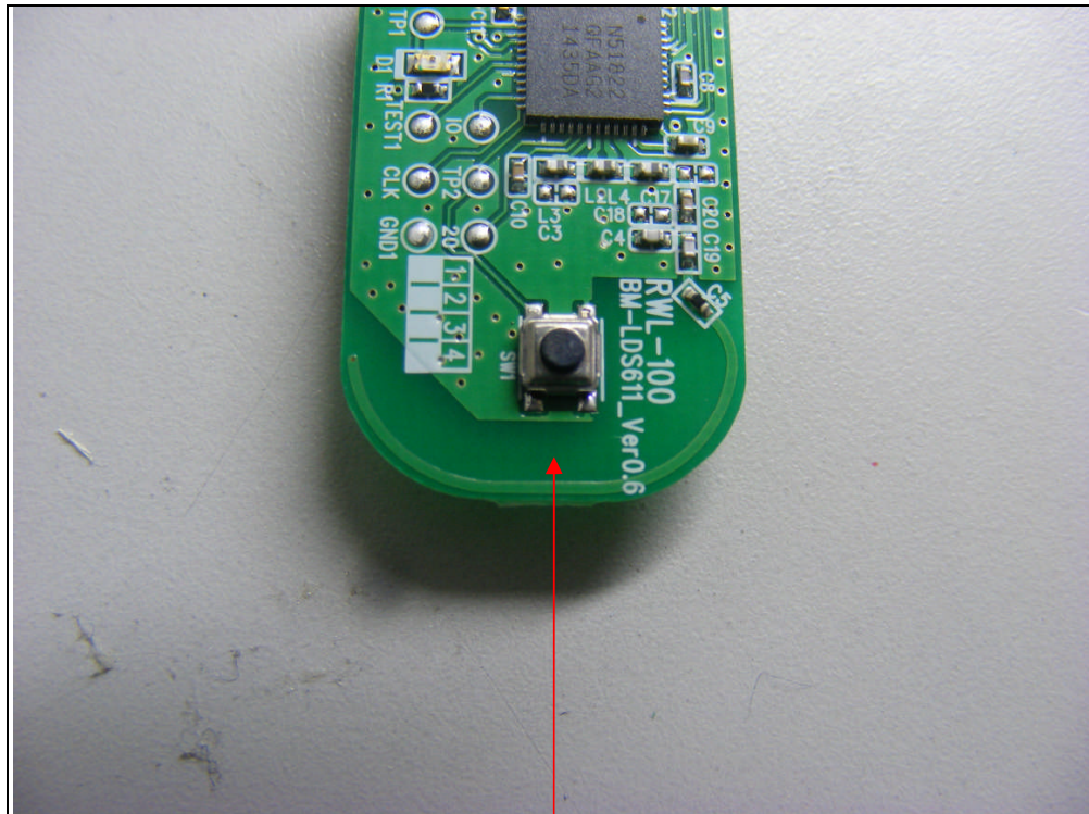
Antenna
