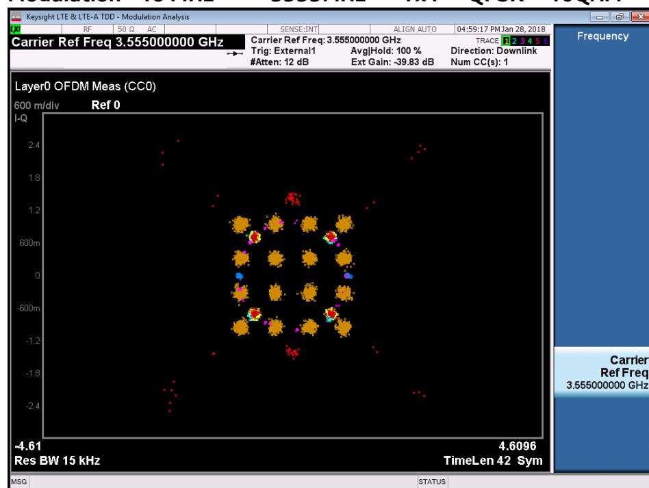
Modulation 10 MHz 3555MHz Tx1 QPSK + 16QAM
