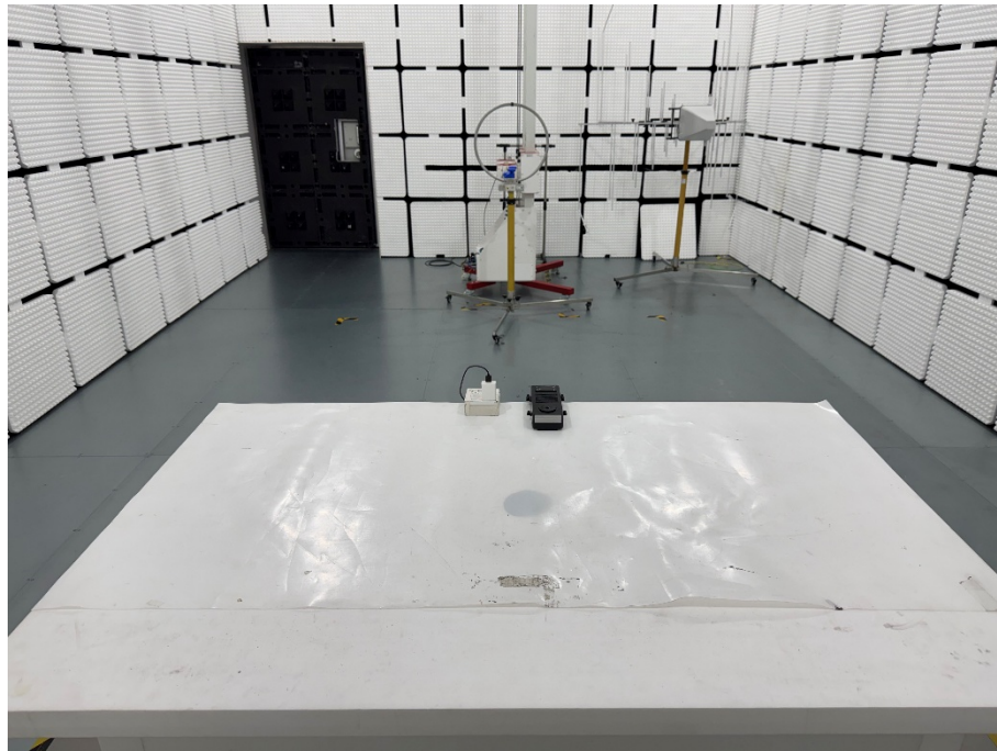
0.009MHz - 30MHz
