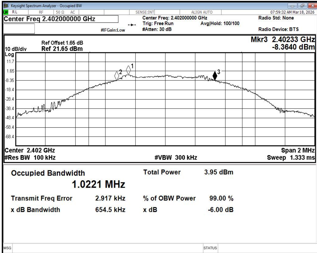
-6dB Bandwidth NVNT BLE 2402MHz Ant1
