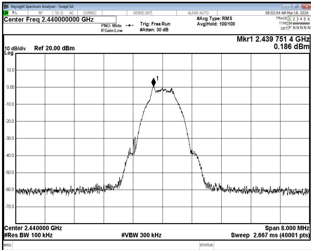
Tx. Spurious NVNT BLE 2440MHz Ant1 Ref
