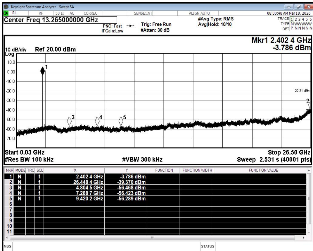
Tx. Spurious NVNT BLE 2402MHz Ant1 Emission
