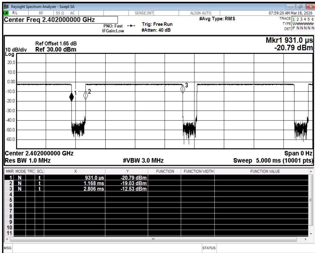
Duty Cycle NVNT BLE 2402MHz Ant1
