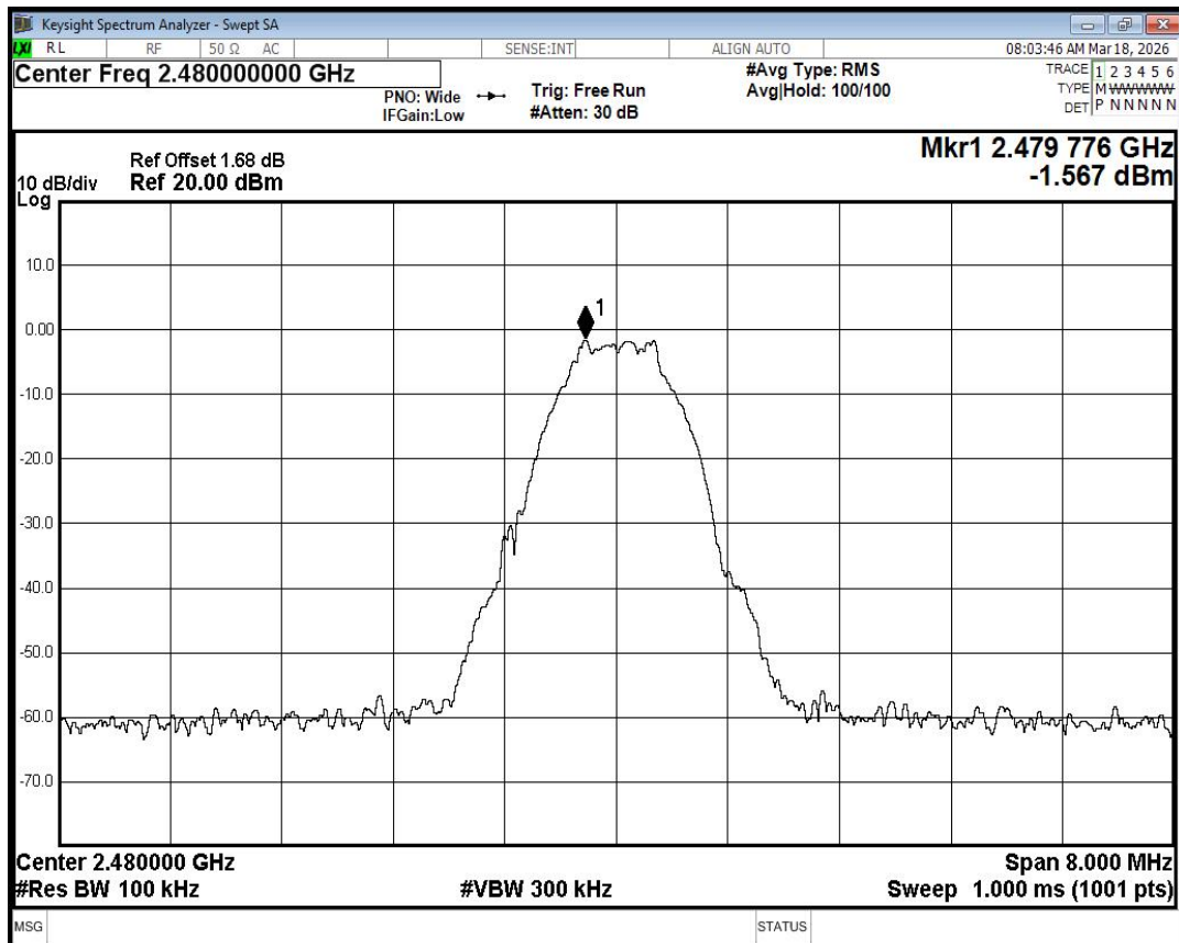
Band Edge NVNT BLE 2480MHz Ant1 Ref
