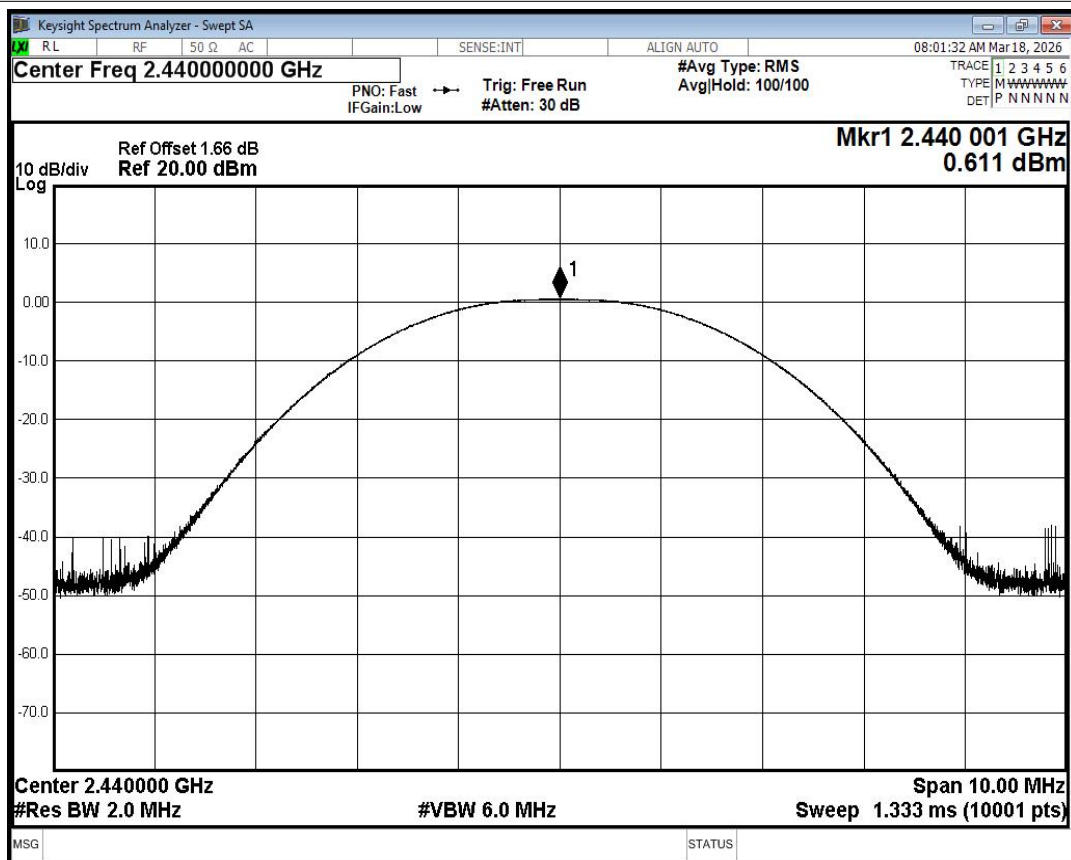
Peak Power NVNT BLE 2440MHz Ant1
