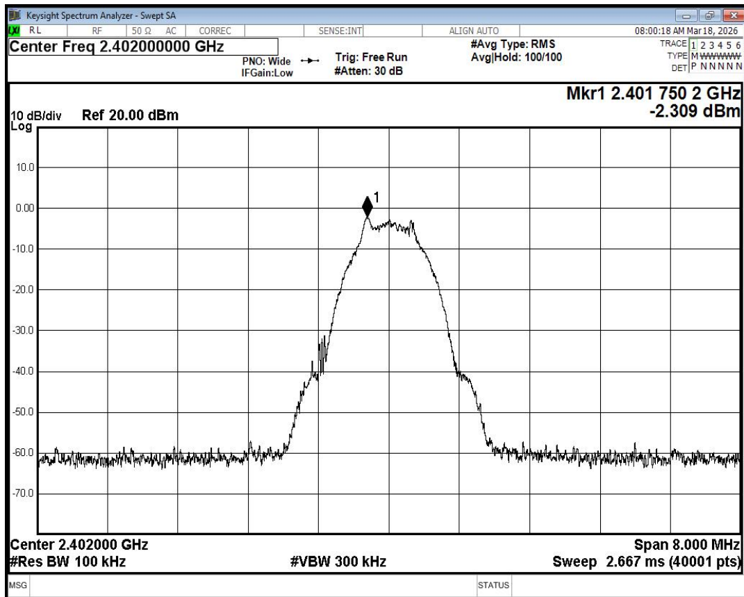
Tx. Spurious NVNT BLE 2402MHz Ant1 Ref
