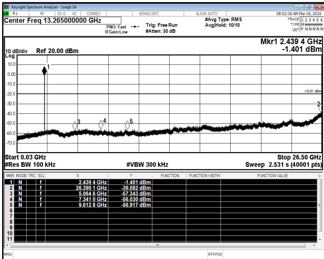
Tx. Spurious NVNT BLE 2440MHz Ant1 Emission
