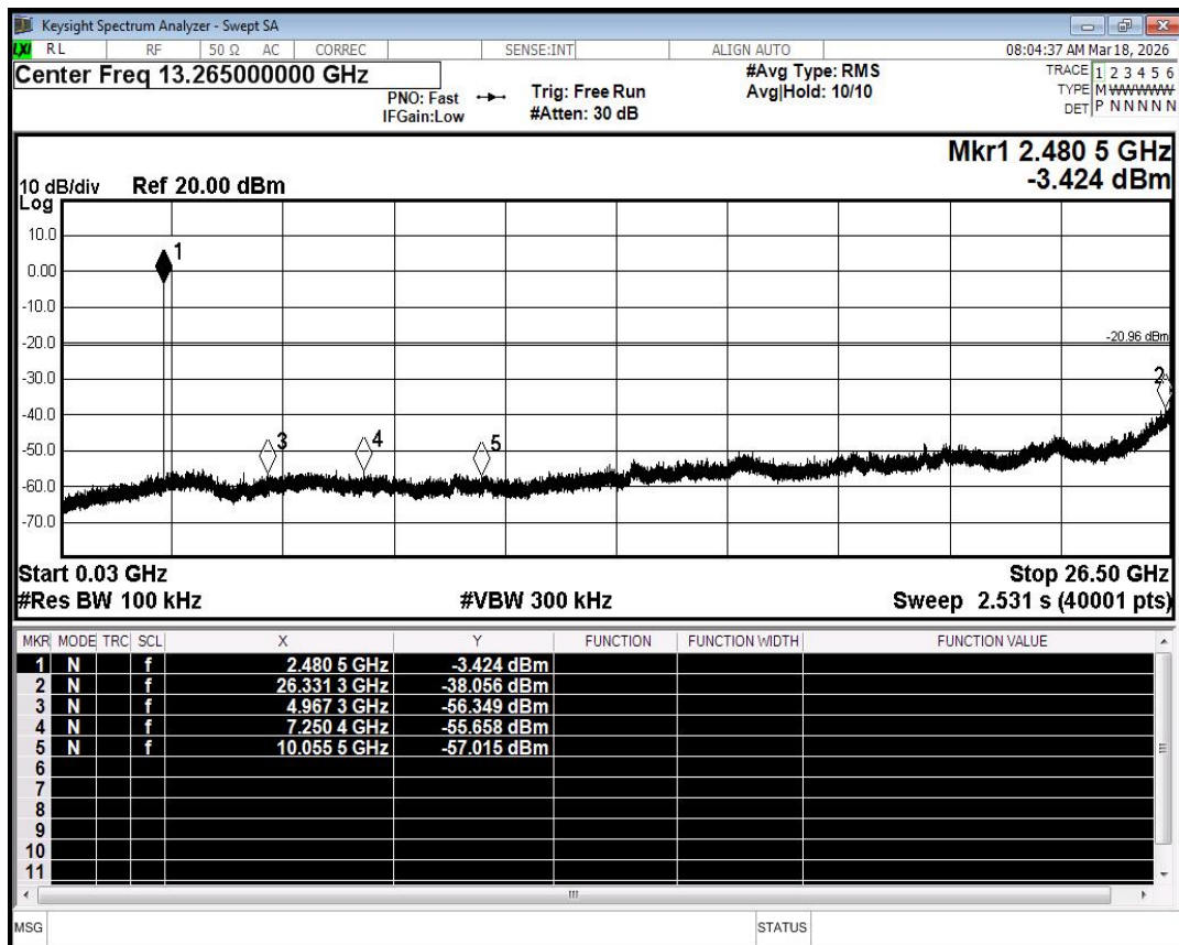
Tx. Spurious NVNT BLE 2480MHz Ant1 Emission
