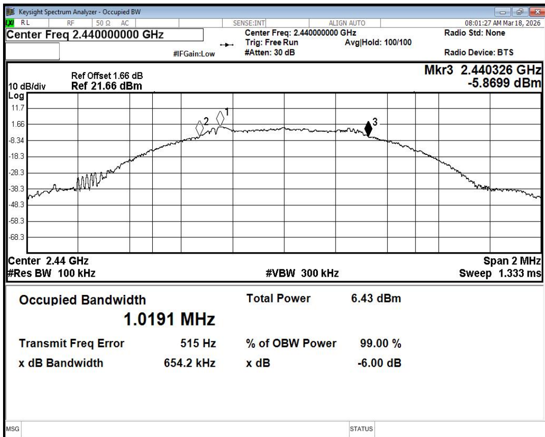
-6dB Bandwidth NVNT BLE 2440MHz Ant1
