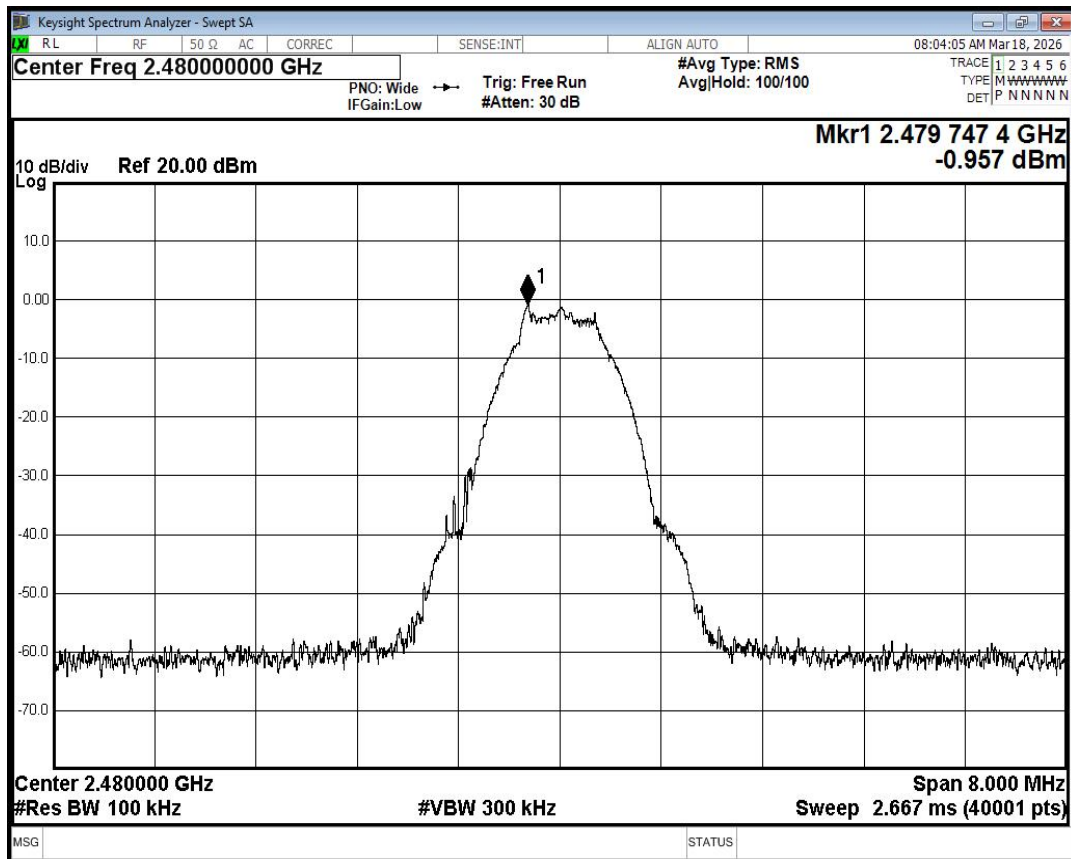
Tx. Spurious NVNT BLE 2480MHz Ant1 Ref
