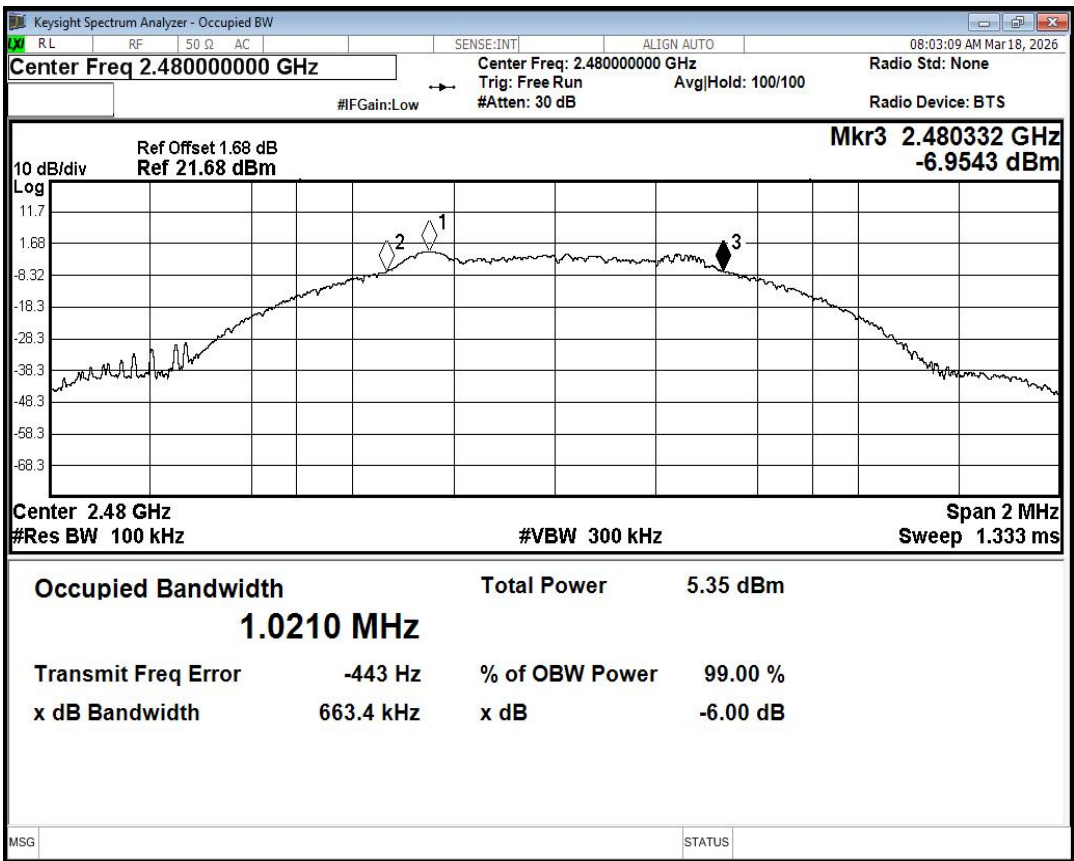
-6dB Bandwidth NVNT BLE 2480MHz Ant1
