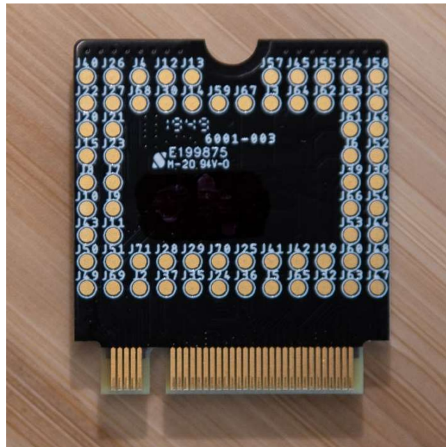
BOTTOM SIDE
