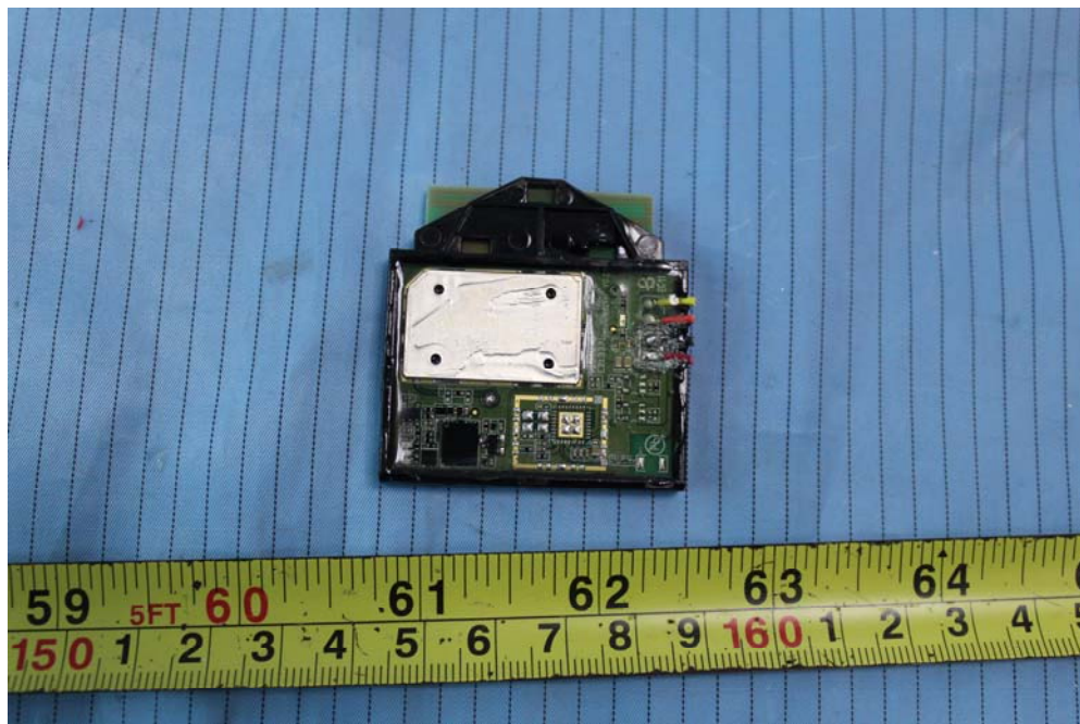
EUT –Module PCB Bottom View
