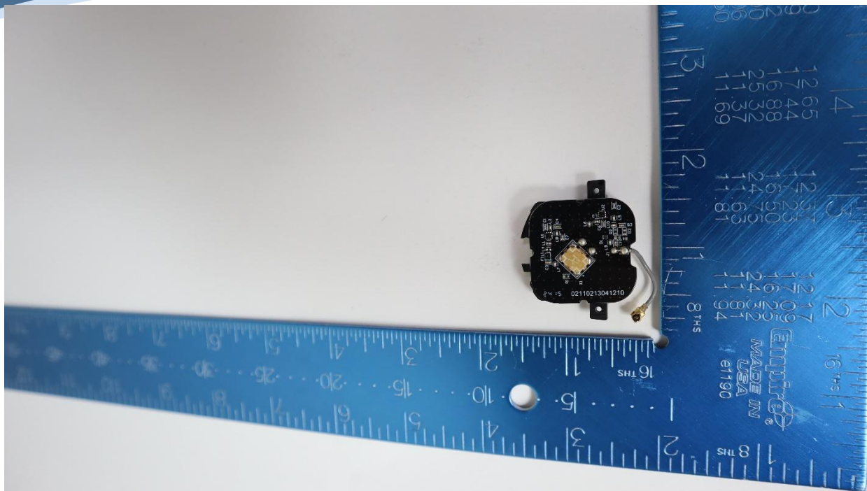
S8 Tag GPS module back
