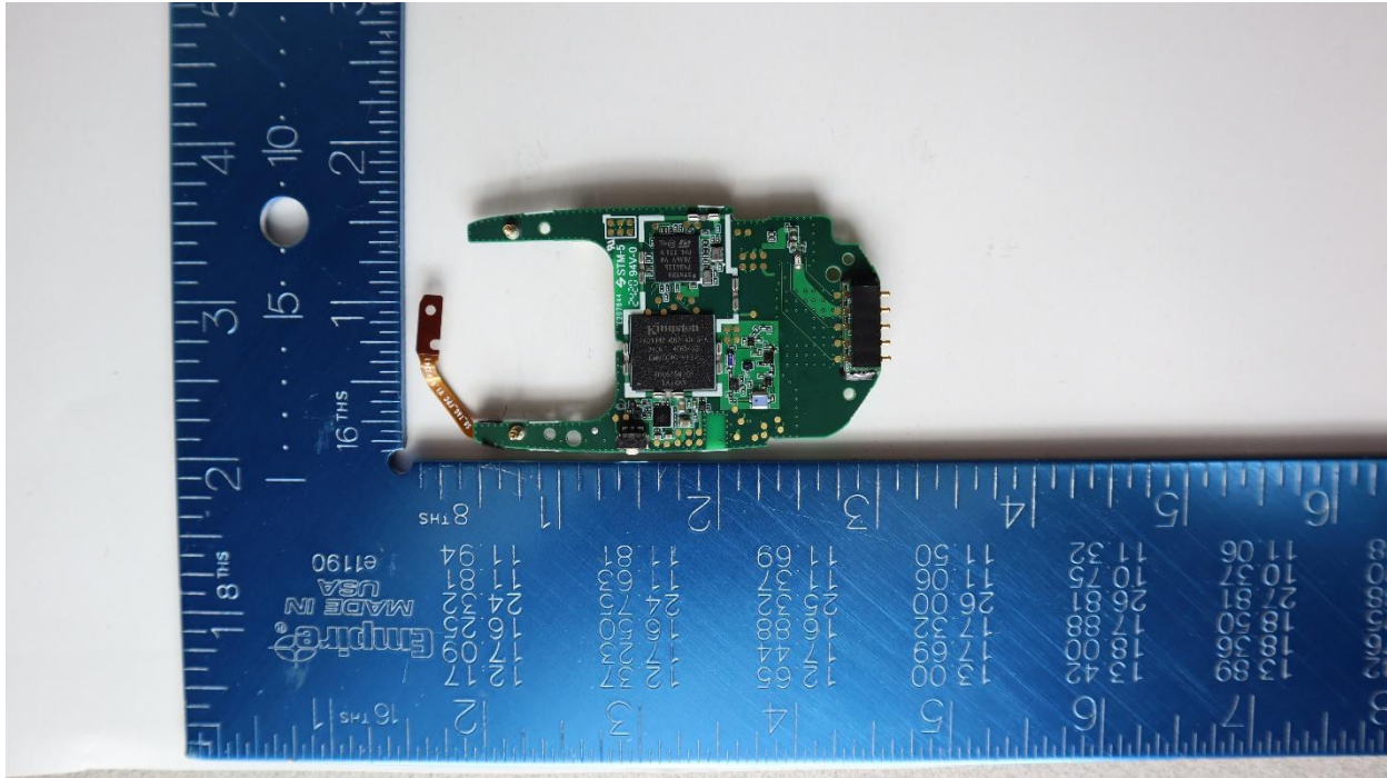
RF module
