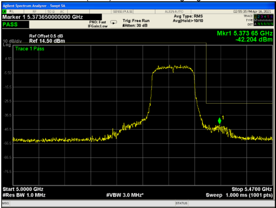
802.11ac(HT80) U-NII-2A Band edge-right side
