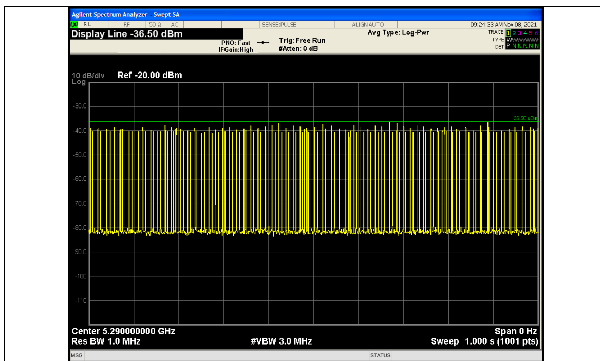
802.11ac(HT80) channel 58 5290MHz
