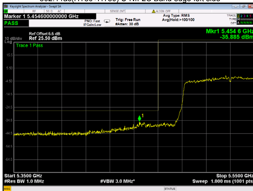
802.11ac(HT80+HT80) U-NII-2C Band edge-left side
