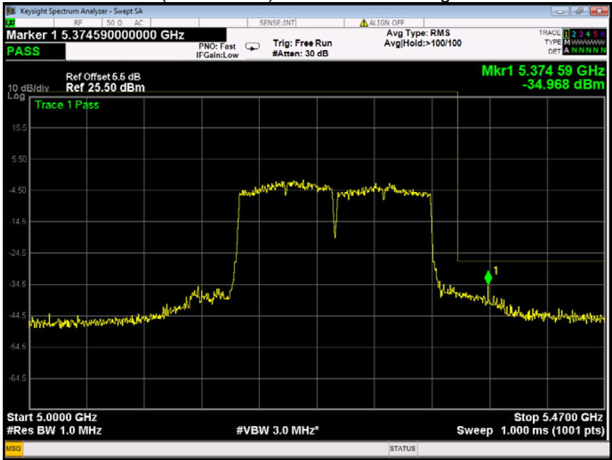
802.11ac(HT80+HT80) U-NII-1/2A Band edge-left side
