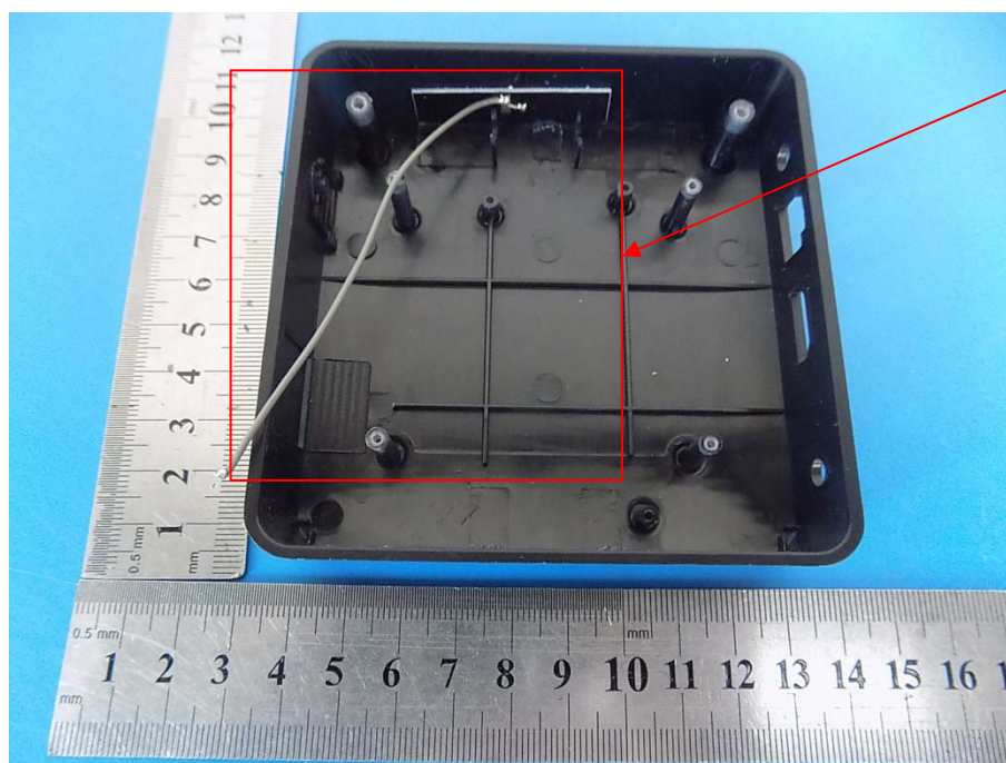
BT/WiFi Antenna
