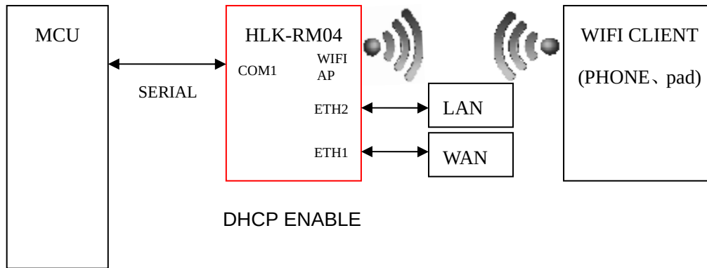
Fig6.4..Default mode model
