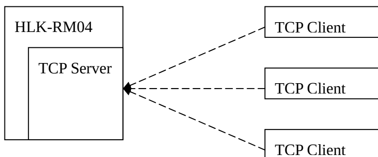
Fig6.4.1.TCP Server
