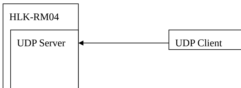
Fig6.4.3.UDP Server
