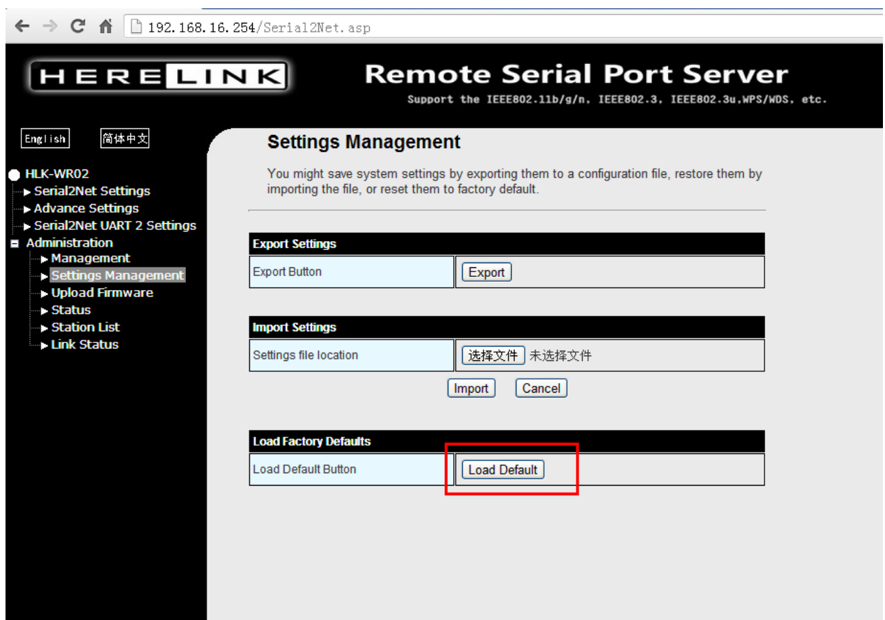
Fig 8-1Load Default
