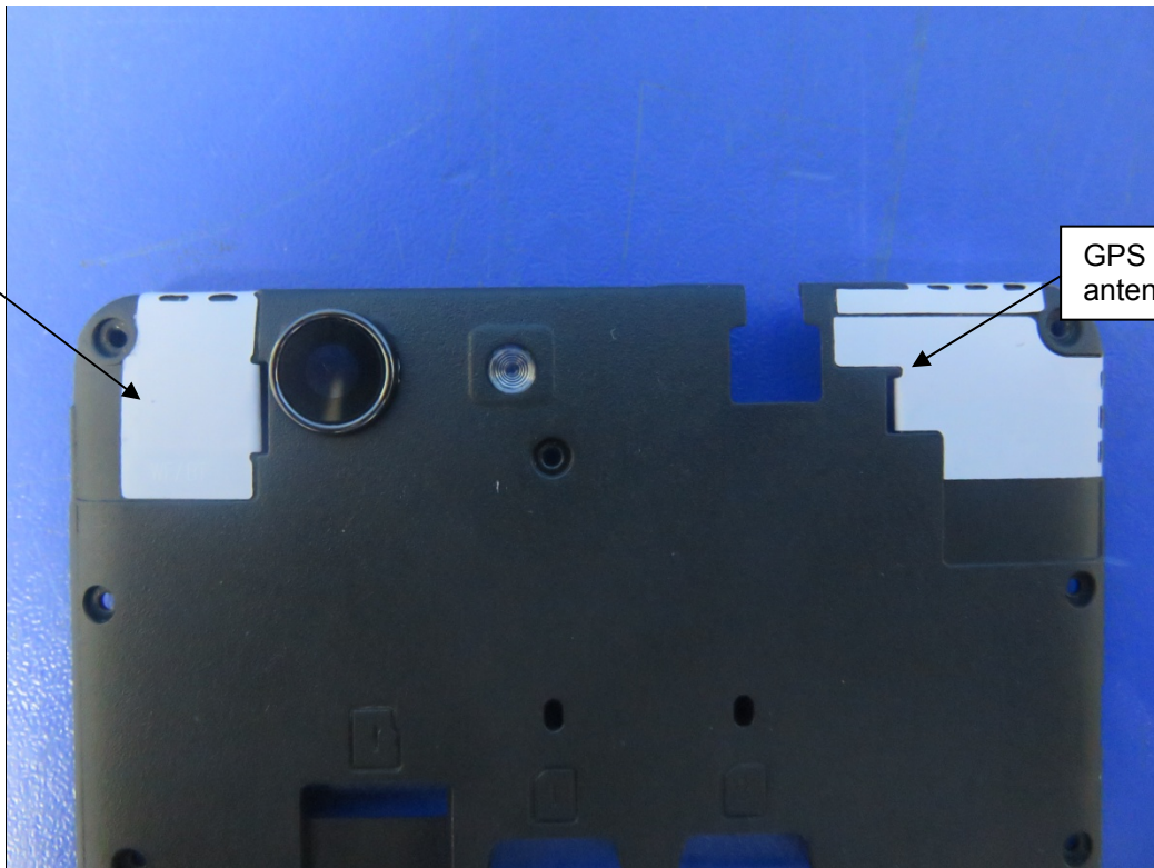
GSM/WCDMA antenna
