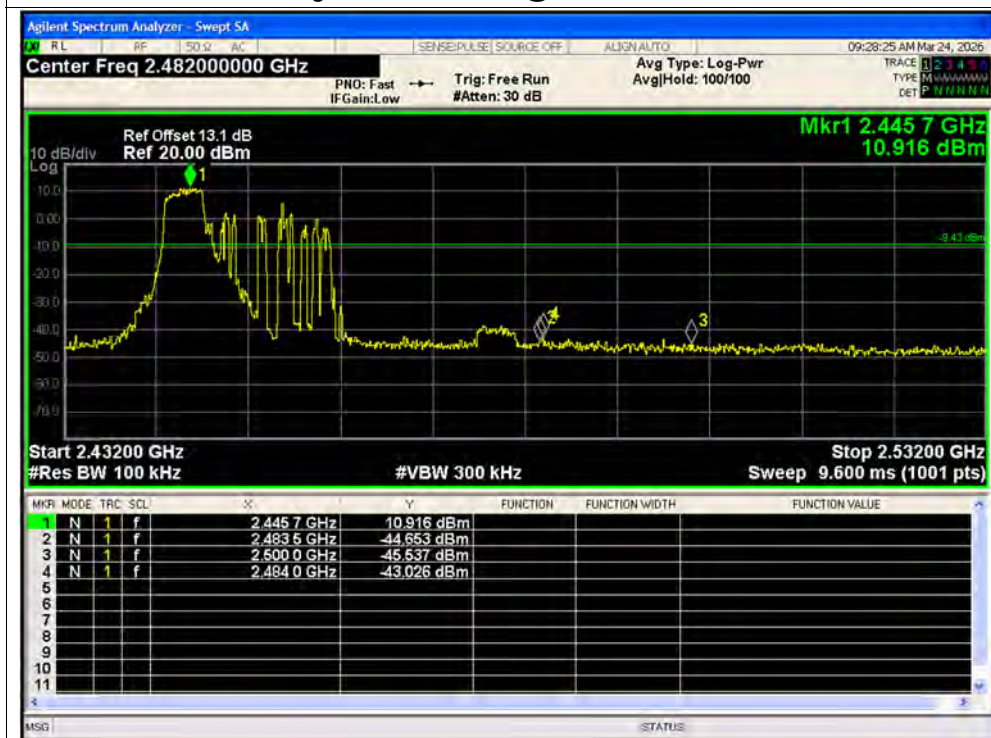
Band Edge NVNT ax40 52@37 2462MHz Ant1 Emission
