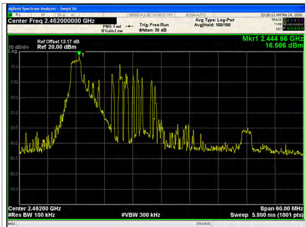
Band Edge NVNT ax40 26@0 2462MHz Ant2 Ref
