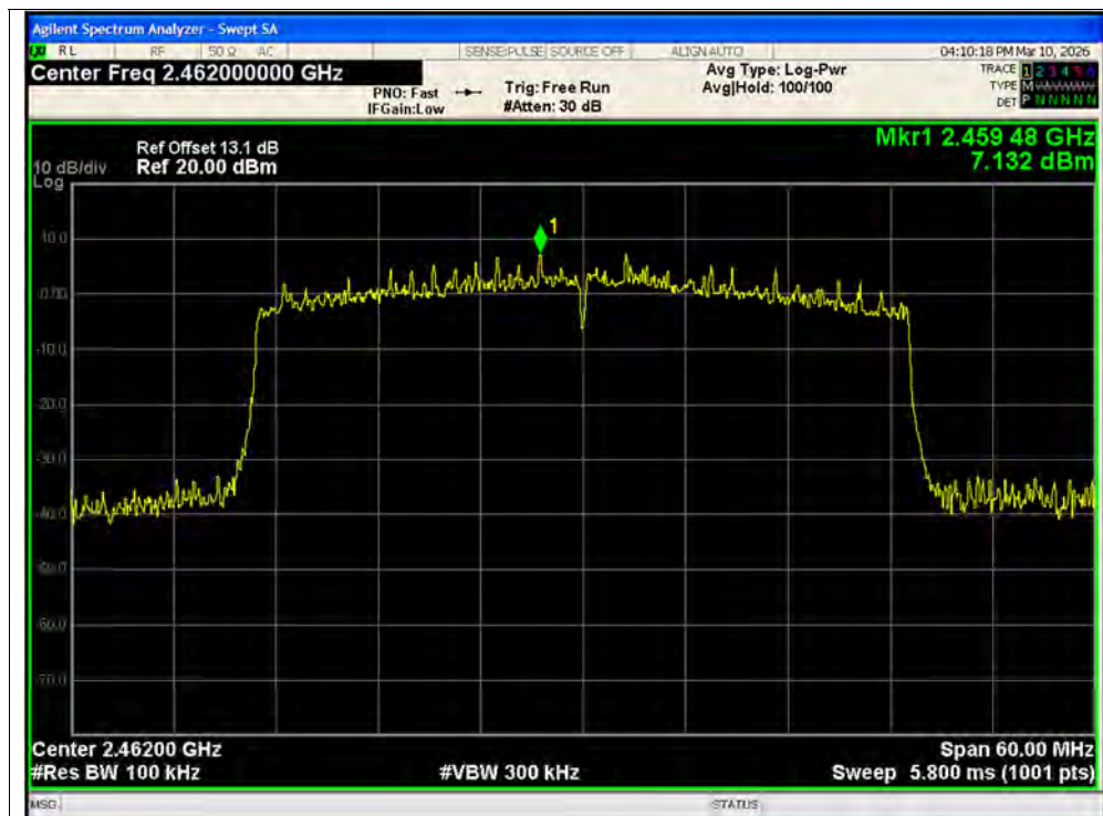
Band Edge NVNT ax40 2462MHz Ant1 Ref
