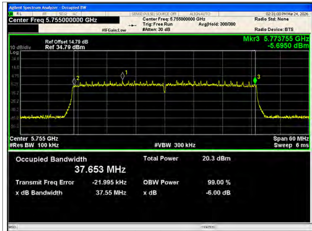
-6dB Bandwidth NVNT ax40 5755MHz Ant1 MIMO
