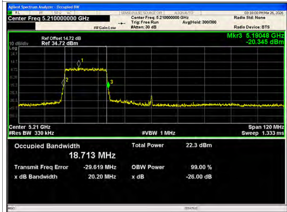
-26dB Bandwidth NVNT ax80 242@1 5210MHz Ant2 MIMO
