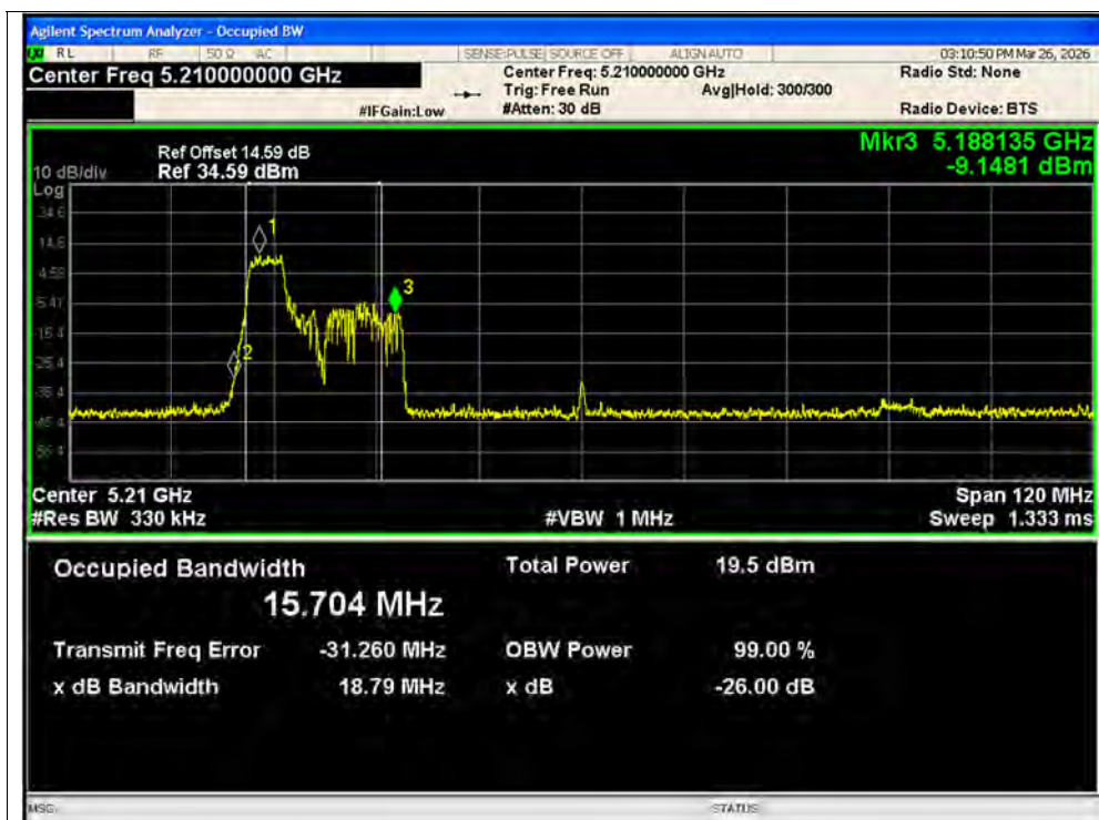
-26dB Bandwidth NVNT ax80 52@1 5210MHz Ant1 MIMO
