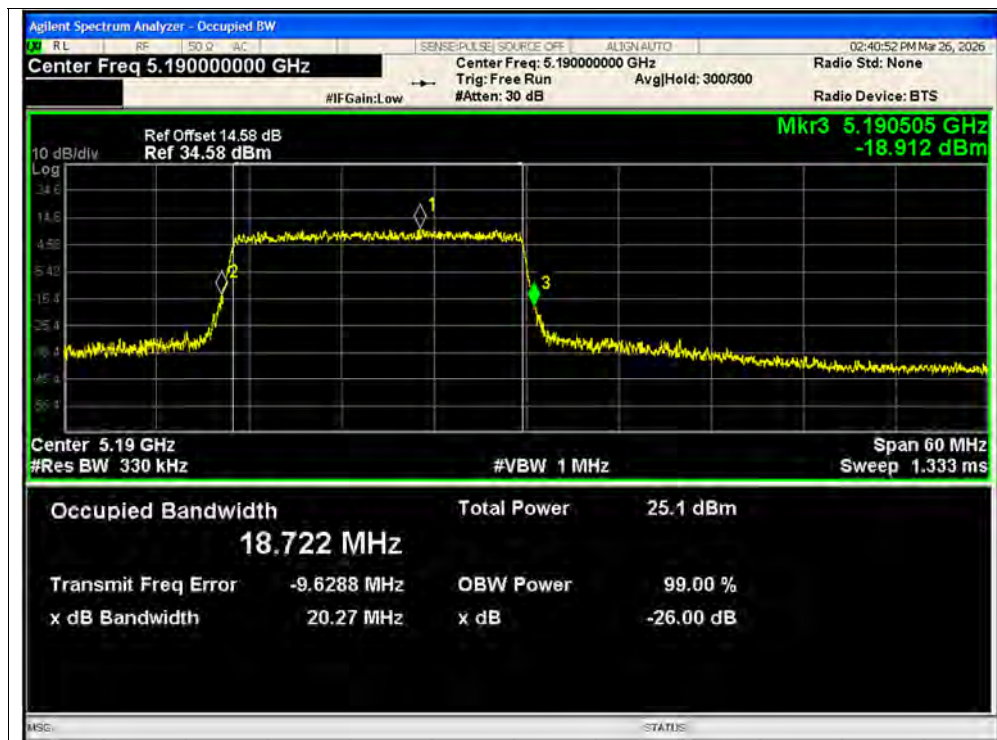
-26dB Bandwidth NVNT ax40 242@1 5190MHz Ant1 MIMO
