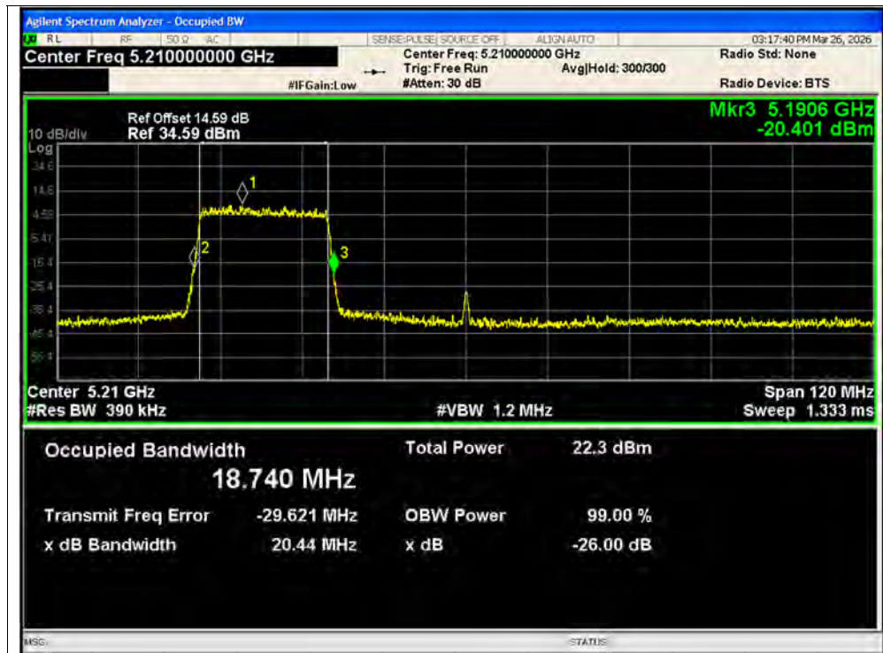
-26dB Bandwidth NVNT ax80 242@1 5210MHz Ant1 MIMO
