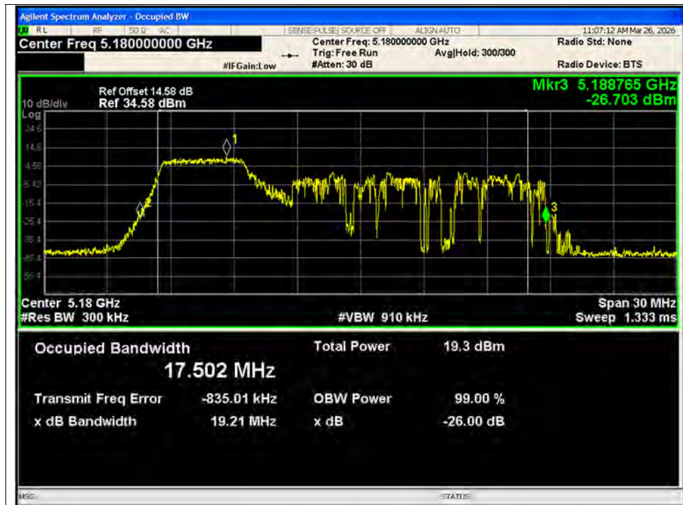
-26dB Bandwidth NVNT ax20 52@1 5180MHz Ant1 MIMO
