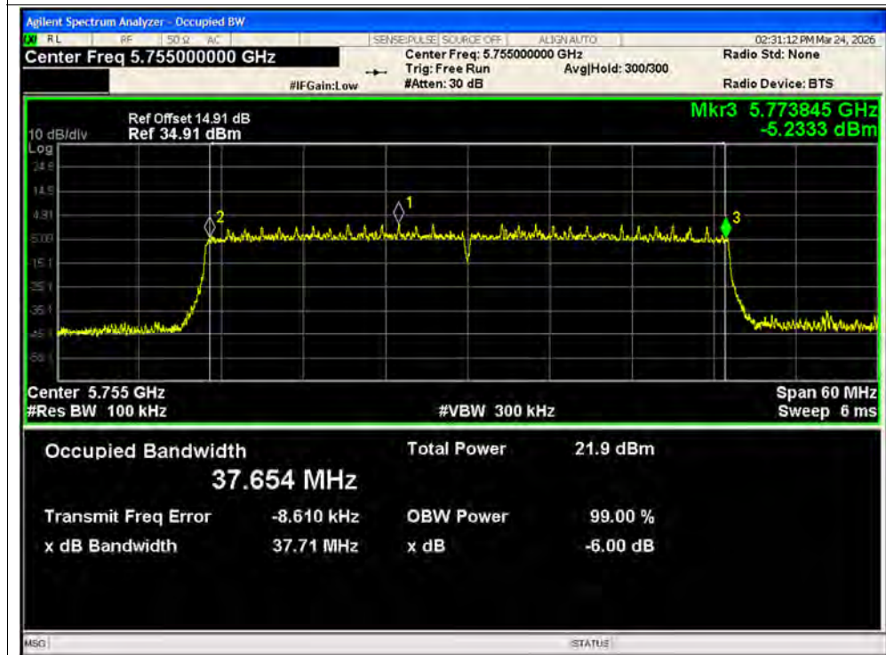
-6dB Bandwidth NVNT ax40 5755MHz Ant2 MIMO
