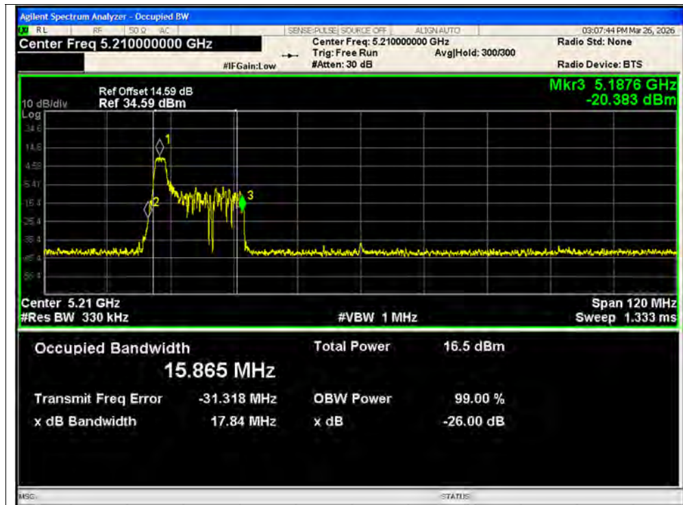
-26dB Bandwidth NVNT ax80 26@1 5210MHz Ant1 MIMO
