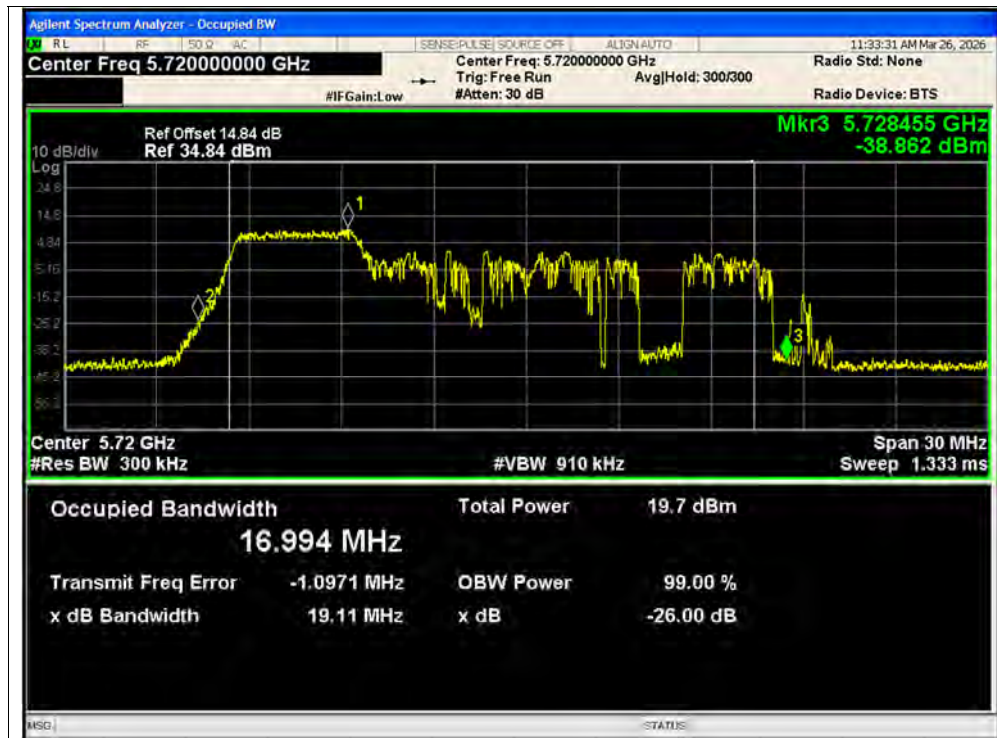
-26dB Bandwidth NVNT ax20 52@1 5720MHz Ant1 MIMO
