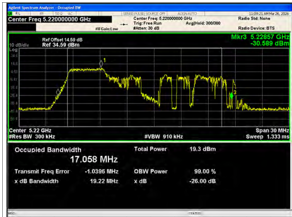
-26dB Bandwidth NVNT ax20 52@1 5220MHz Ant1 MIMO
