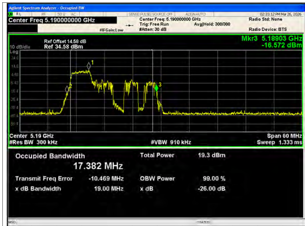
-26dB Bandwidth NVNT ax40 52@1 5190MHz Ant1 MIMO
