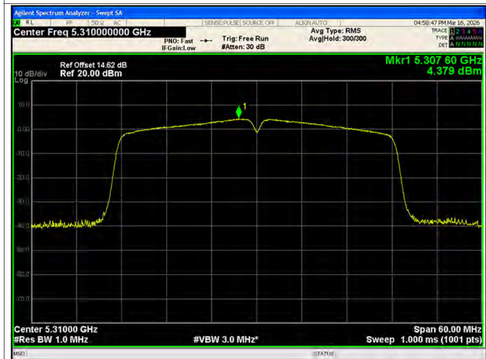
PSD NVNT n40 5310MHz Ant1 SISO
