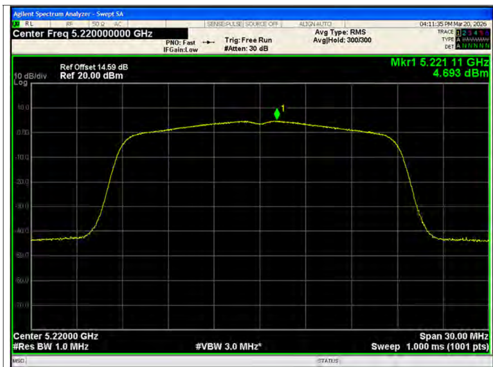
PSD NVNT ac20 5220MHz Ant1 MIMO
