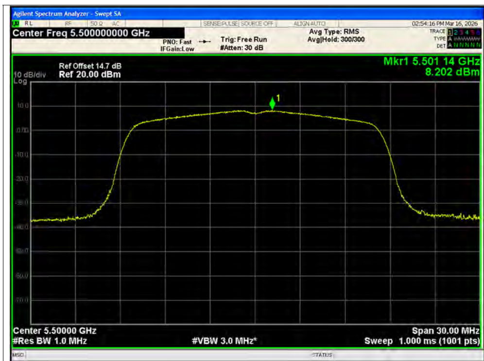
PSD NVNT a 5500MHz Ant1 SISO
