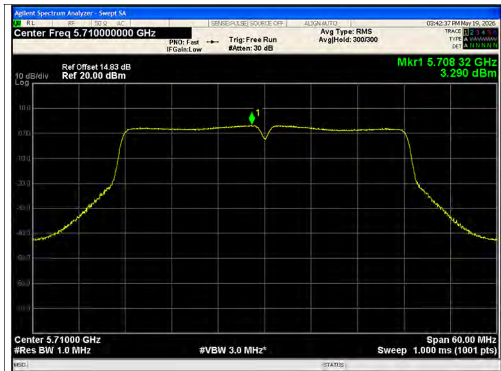
PSD NVNT n40 5710MHz Ant1 SISO
