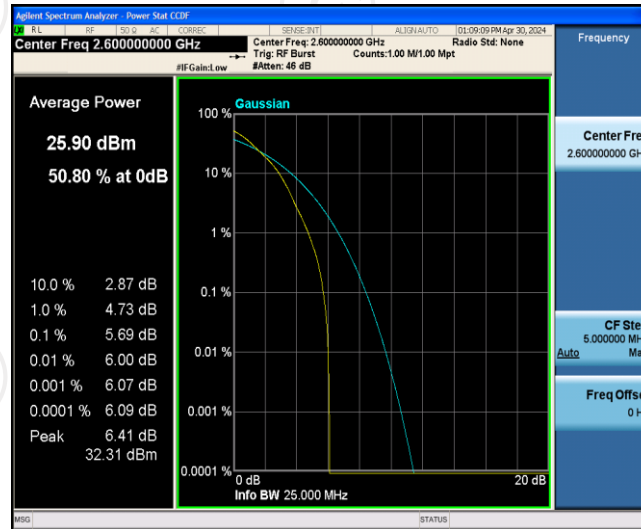
Band41-20MHz-QPSK-40690-1RB#0
