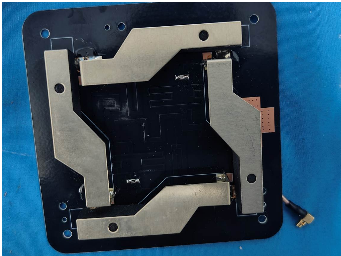
RFID Antenna
