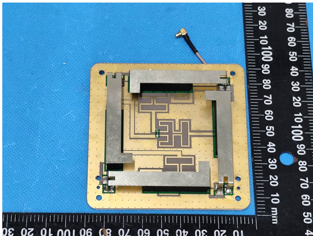
RFID Antenna
