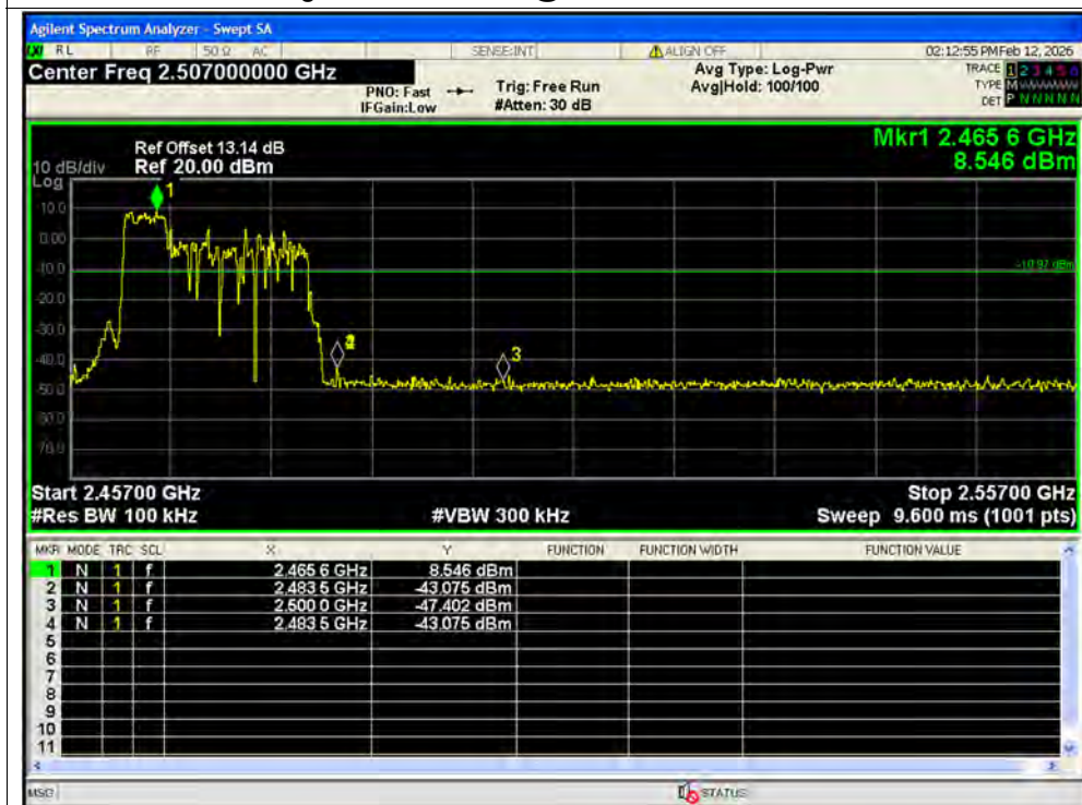
Band Edge NVNT ax20 52@37 2472MHz Ant1 Emission SISO
