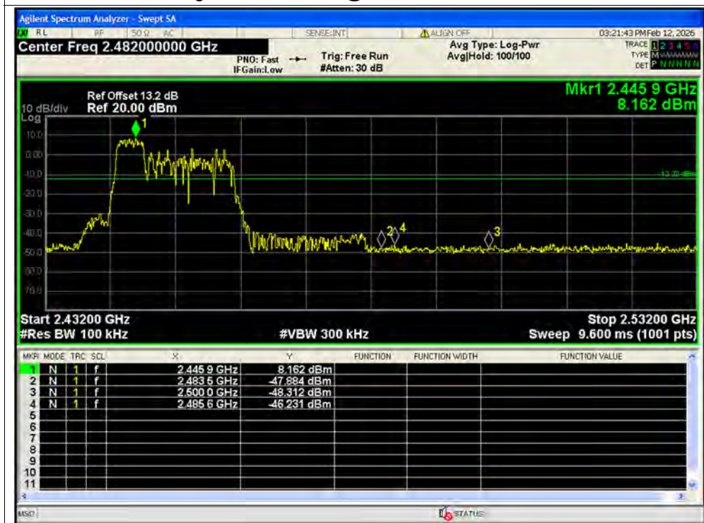
Band Edge NVNT ax40 52@37 2462MHz Ant1 Emission SISO
