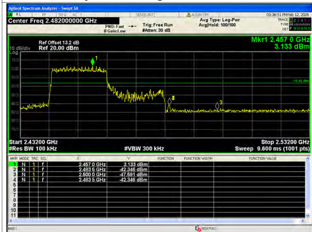
Band Edge NVNT ax40 242@61 2462MHz Ant1 Emission SISO
