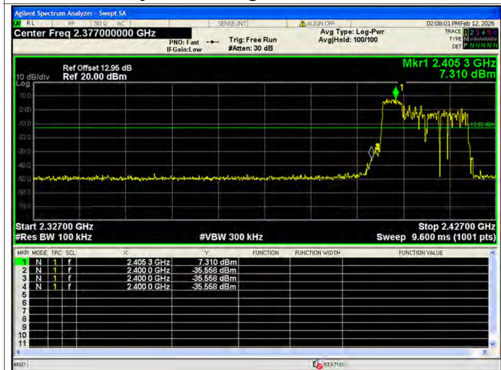
Band Edge NVNT ax20 52@37 2412MHz Ant1 Emission SISO
