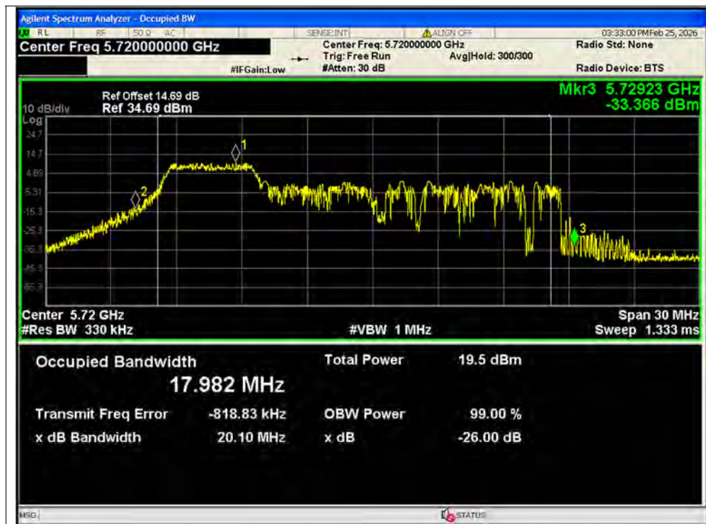
-26dB Bandwidth NVNT ax20 52@1 5720MHz Ant1 MIMO
