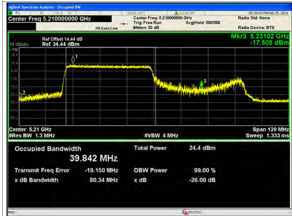
-26dB Bandwidth NVNT ax80 484@1 5210MHz Ant2 MIMO
