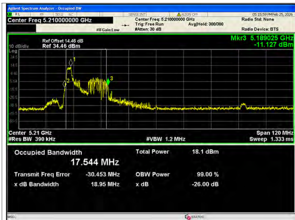
-26dB Bandwidth NVNT ax80 26@1 5210MHz Ant1 MIMO
