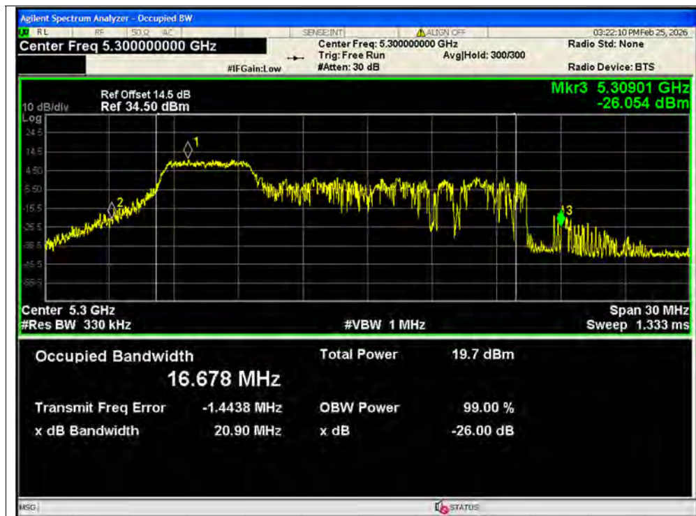
-26dB Bandwidth NVNT ax20 52@1 5300MHz Ant1 MIMO
