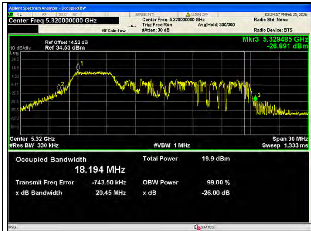
-26dB Bandwidth NVNT ax20 52@1 5320MHz Ant1 MIMO
