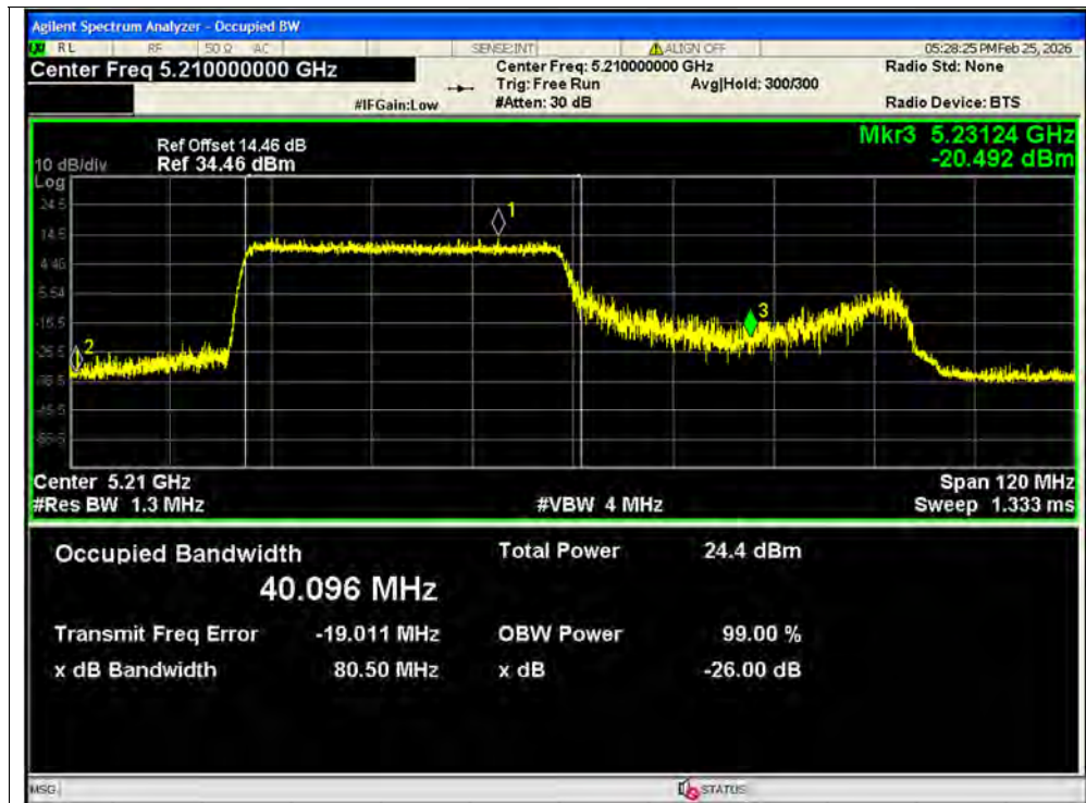
-26dB Bandwidth NVNT ax80 484@1 5210MHz Ant1 MIMO
