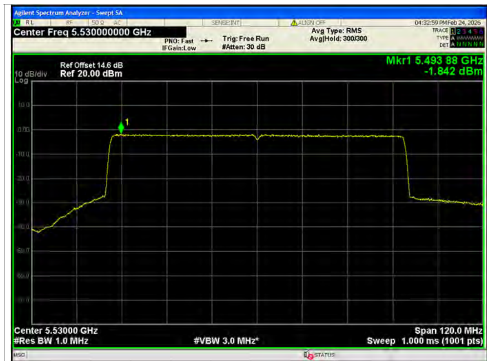
PSD NVNT ax80 5530MHz Ant1 MIMO
