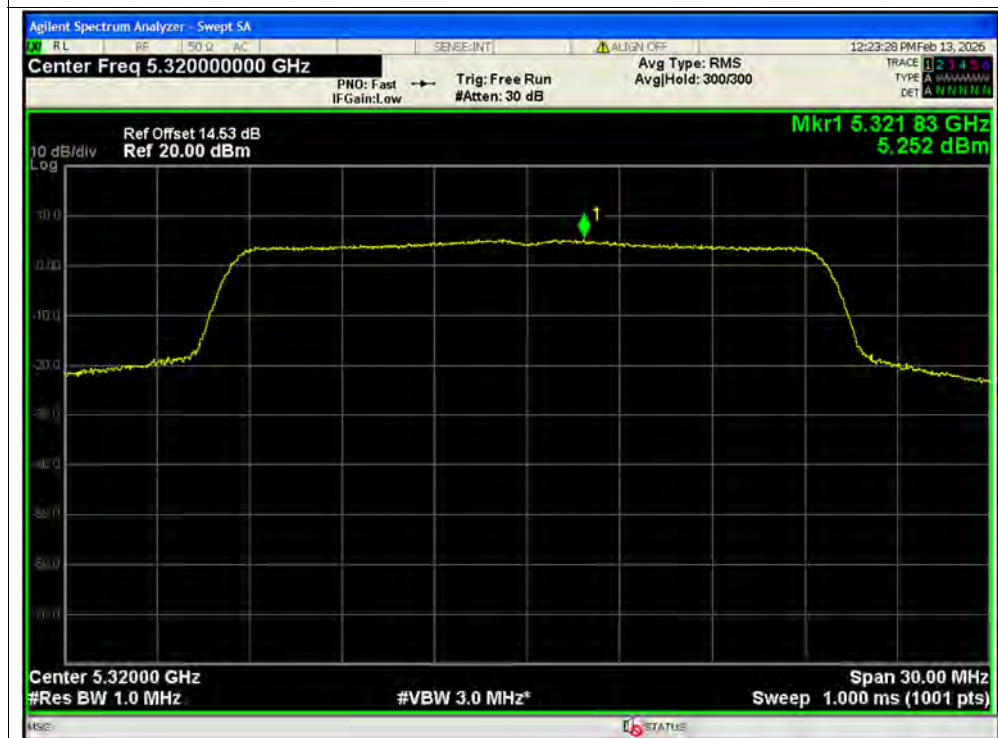
PSD NVNT ax20 5320MHz Ant1 SISO
