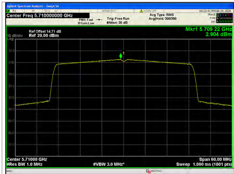
PSD NVNT ax40 5710MHz Ant1 MIMO
