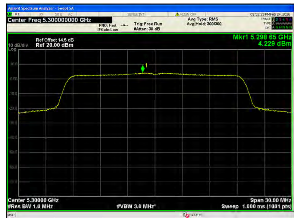
PSD NVNT ax20 5300MHz Ant1 MIMO
