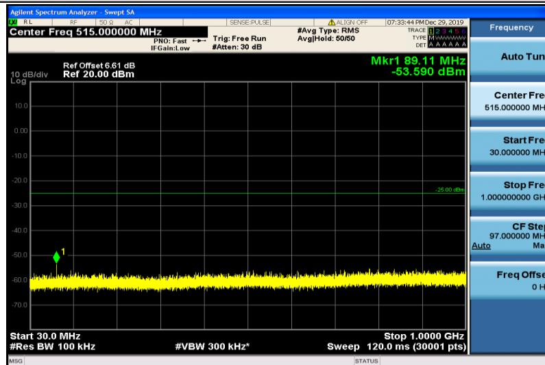
Band41-5MHz-QPSK-41215-1RB#0-30~1000MHz
