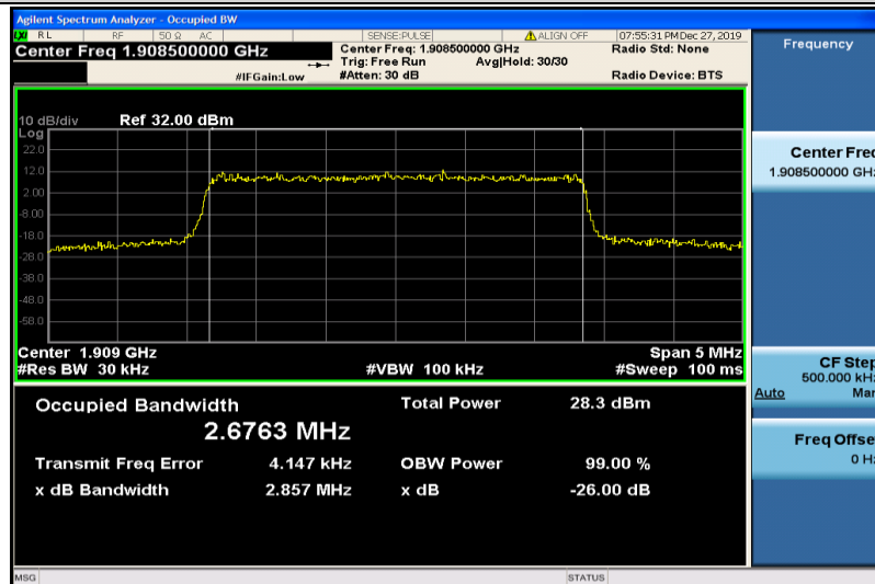
Band2-3MHz-QPSK-19185-15RB#0-2.6763
