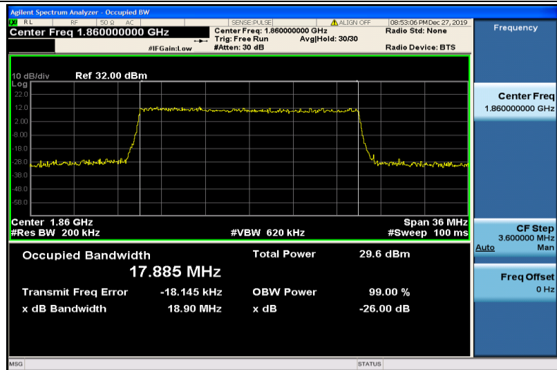
Band2-20MHz-QPSK-18700-100RB#0-17.885
