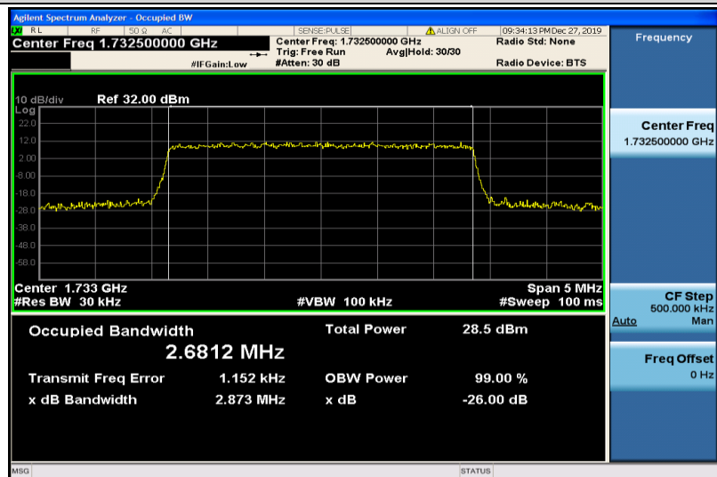
Band4-3MHz-QPSK-17325-15RB#0-2.6812
