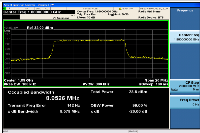
Band2-10MHz-QPSK-18900-50RB#0-8.9526
