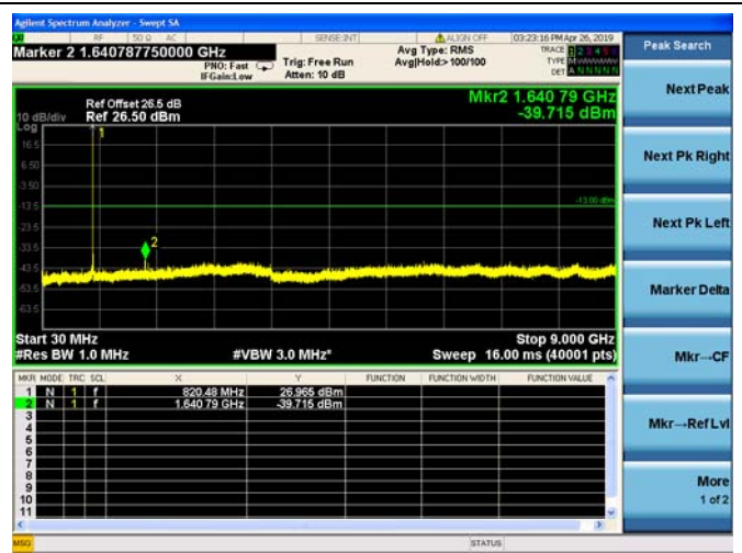
FDD18_MiddleRange_1.4MHz_30MHz~9GHz 16QAM
