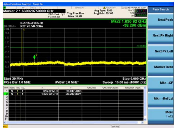
FDD18_MiddleRange_1.4MHz_30MHz~9GHz 16QAM
