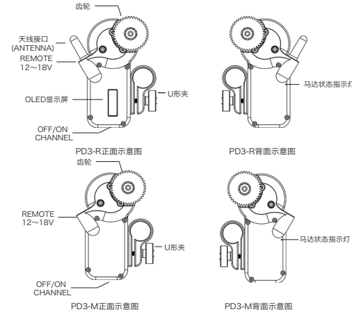
马达示意图
