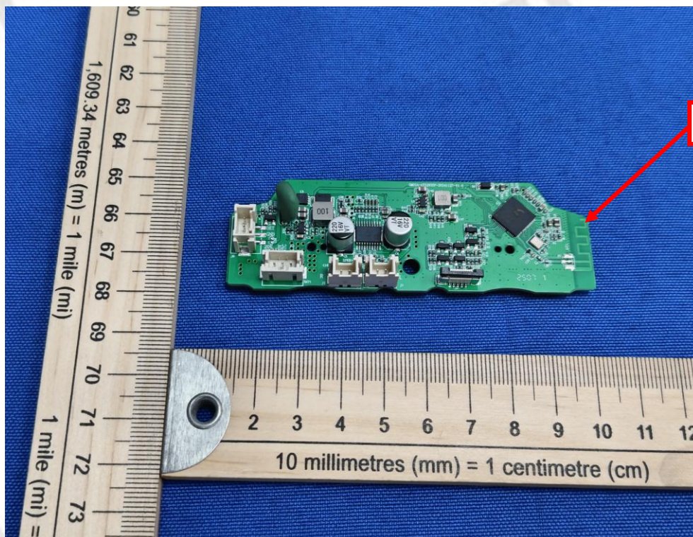
BLE Antenna
