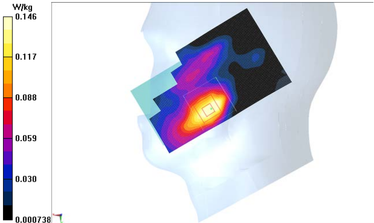
Fig.11 LTE Band2
