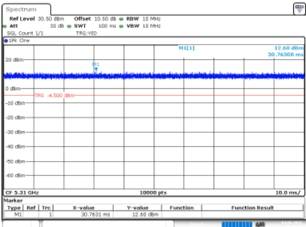
802.11n40_5310MHz
