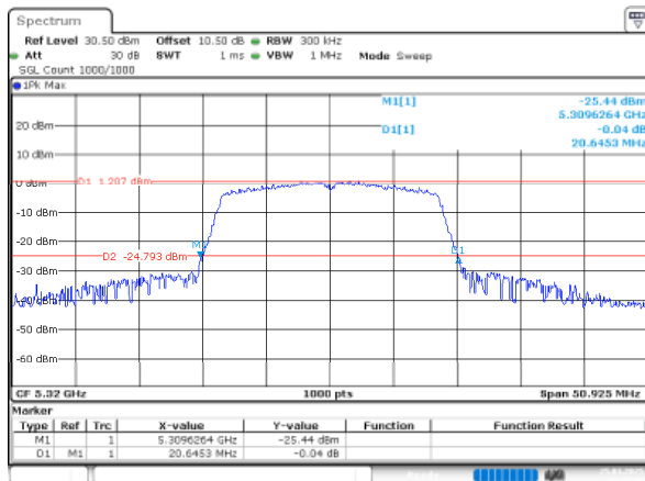
802.11n20_5320MHz
