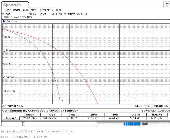
10MHz_Middle_16QAM_50@0
