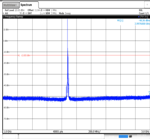
Band25-10MHz-QPSK-26365-1RB#0-1000~3000-PASS
