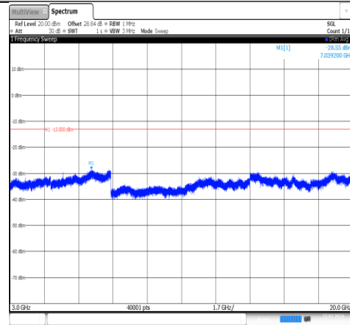
Band25-10MHz-QPSK-26365-1RB#0-3000~20000-PASS
