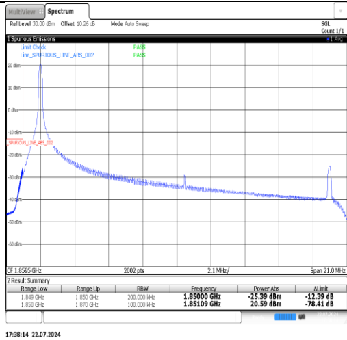
Band25-20MHz-QPSK-26140-1RB#99-PASS
