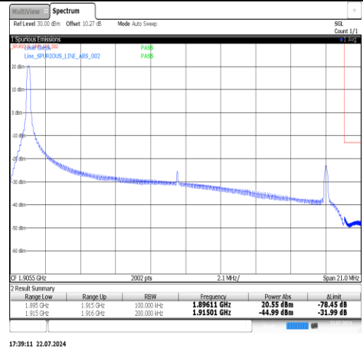
Band25-20MHz-QPSK-26590-1RB#99-PASS
