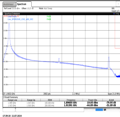
Band25-20MHz-16QAM-26590-1RB#99-PASS
