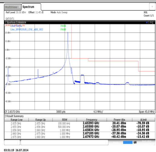
Band41(2535-2655)-20MHz-16QAM-41140-1RB#99-PASS
