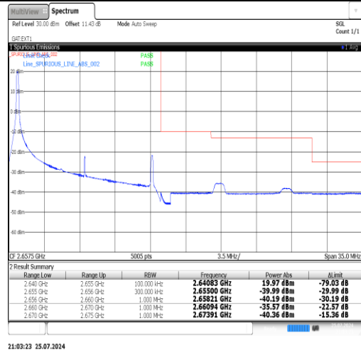
Band41(2535-2655)-15MHz-QPSK-41165-1RB#74-PASS
