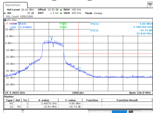
n20_2462MHz_Chain 0
