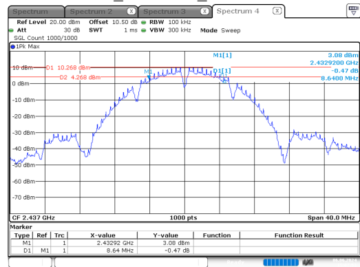
b_2437MHz_Chain 0
