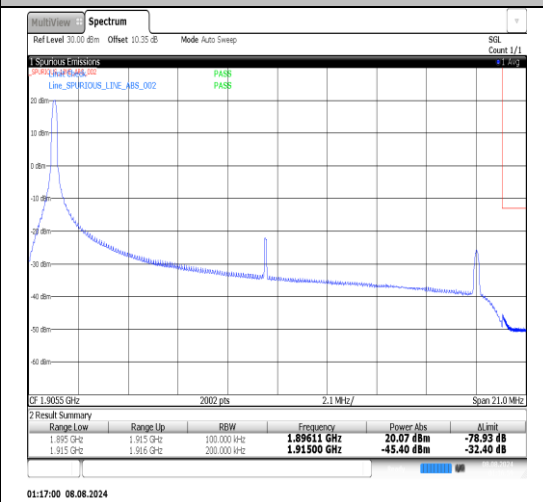
Band25-20MHz-QPSK-26590-1RB#99-PASS
