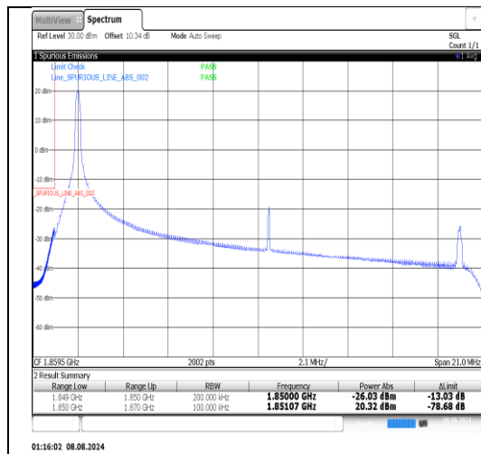
Band25-20MHz-QPSK-26140-1RB#99-PASS
