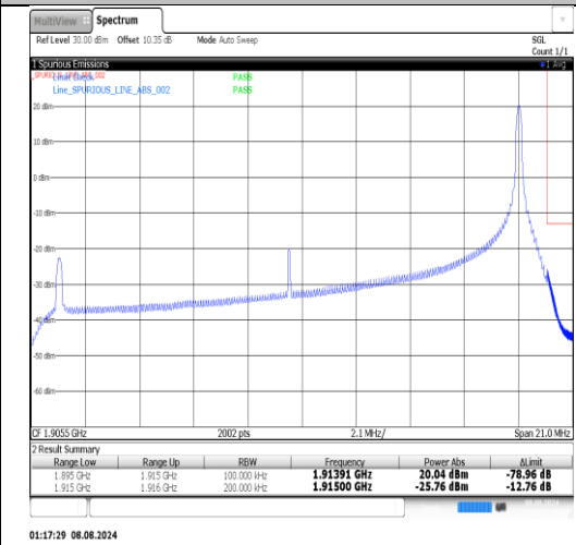
Band25-20MHz-16QAM-26590-1RB#99-PASS
