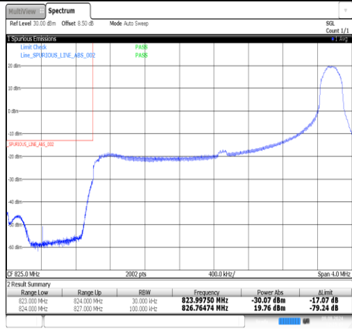
Band26(824-849)-3MHz-QPSK-27025-15RB#0-PASS
