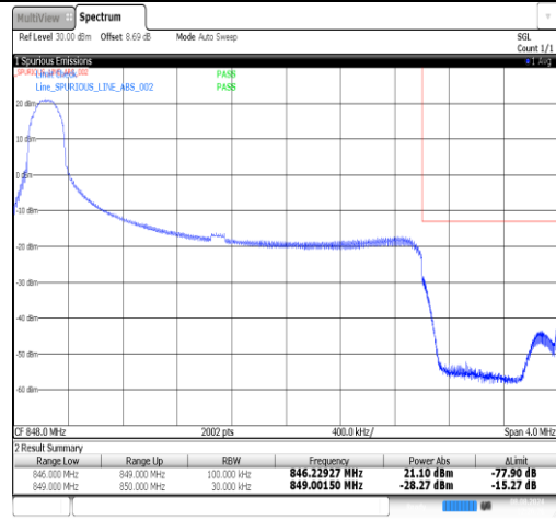
Band26(824-849)-3MHz-QPSK-27025-1RB#14-PASS
