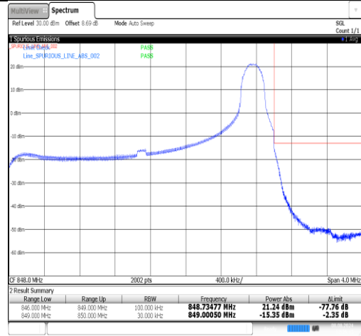
Band26(824-849)-3MHz-QPSK-27025-1RB#14-PASS
