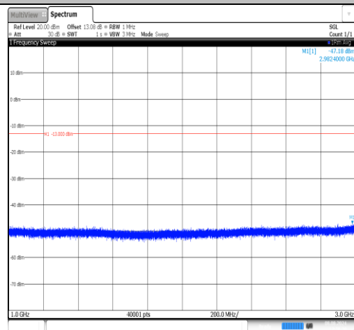
Band26(824-849)-10MHz-QPSK-26840-1RB#0- 1000~3000-PASS
