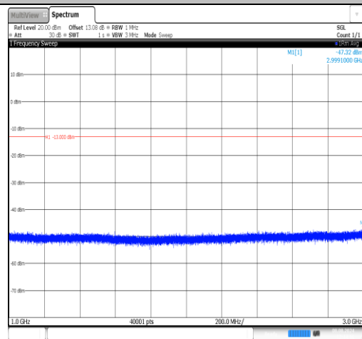
Band26(824-849)-15MHz-QPSK-26865-1RB#0- 1000~3000-PASS
