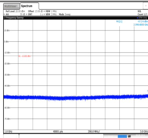
Band26(824-849)-3MHz-16QAM-26915-1RB#0- 1000~3000-PASS
