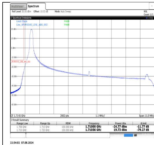
Band4-10MHz-QPSK-20000-1RB#49-PASS
