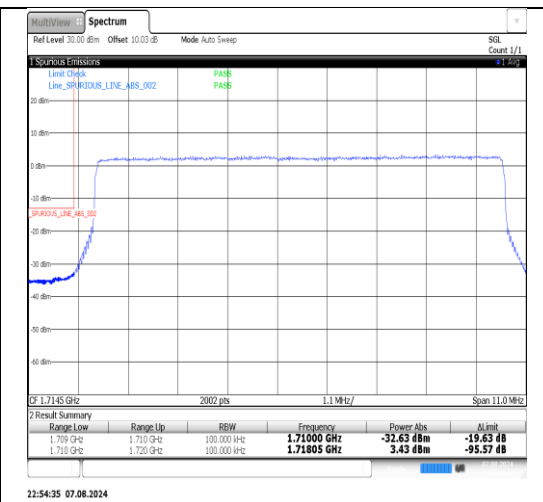
Band4-10MHz-QPSK-20350-1RB#0-PASS
