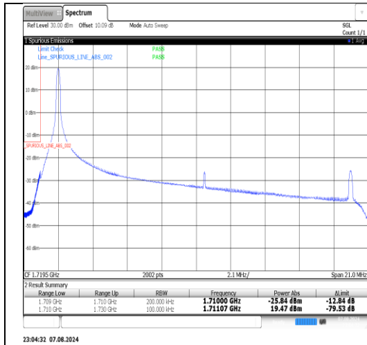
Band4-20MHz-16QAM-20050-1RB#99-PASS
