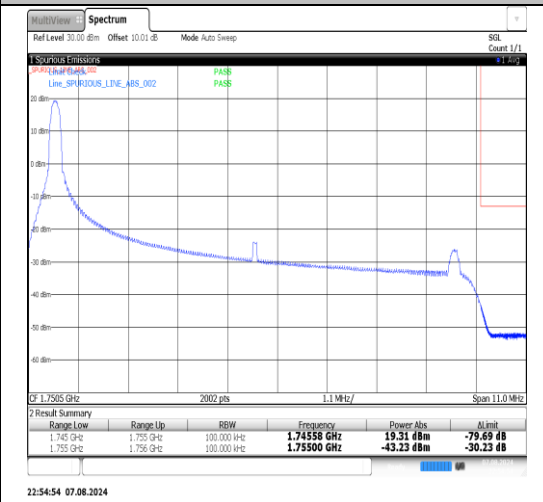
Band4-10MHz-QPSK-20350-1RB#49-PASS
