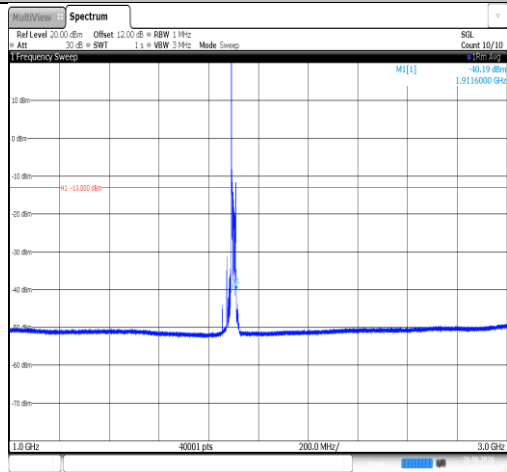
Band2-20MHz-QPSK-19100-1RB#0-1000~3000-PASS
