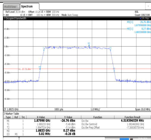
Band25-5MHz-QPSK-26365-25RB#0-PASS
