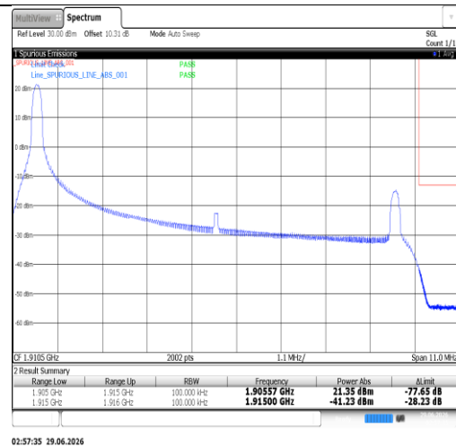
Band25-10MHz-QPSK-26640-50RB#0-PASS
