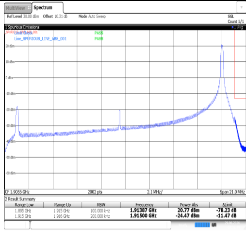
Band25-20MHz-16QAM-26590-1RB#99-PASS
