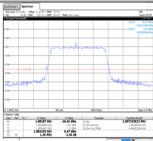
Band25-1.4MHz-QPSK-26365-6RB#0-PASS
