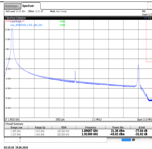
Band25-20MHz-QPSK-26590-100RB#0-PASS
