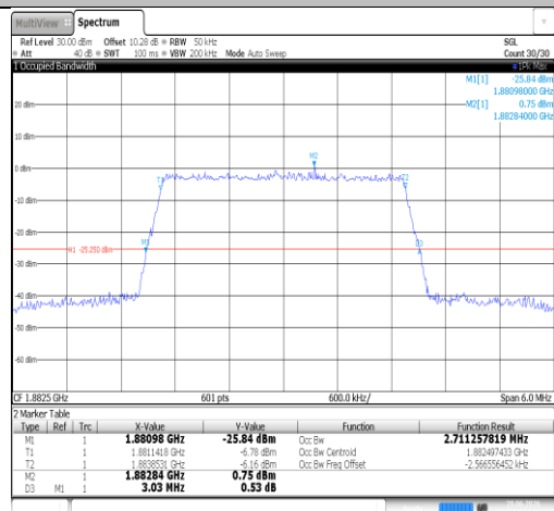
Band25-3MHz-QPSK-26365-15RB#0-PASS
