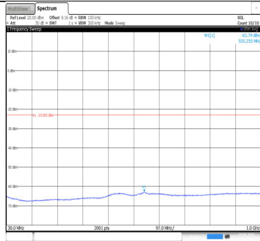
Band25-20MHz-QPSK-26365-1RB#0-30~1000-PASS
