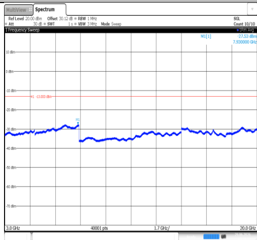
Band25-15MHz-QPSK-26115-1RB#0-3000~20000-PASS
